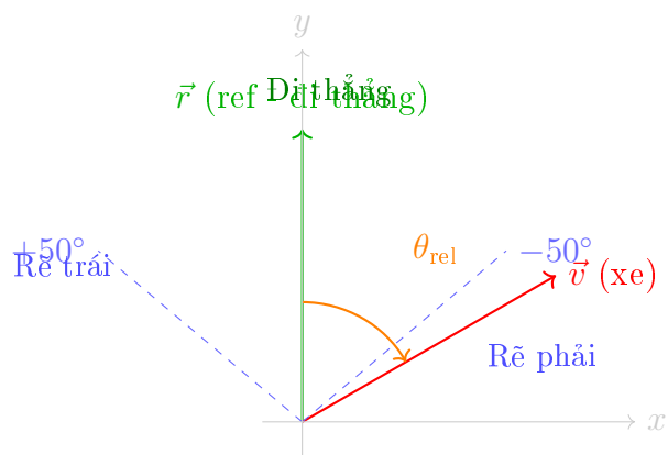
Hình 2.4: So sánh góc chuyển động \vec{v} với góc tham chiếu \vec{r} (ngưỡng 50^\circ ). Vùng màu xanh lá: đi thẳng, vùng ngoài: rẽ trái/phải.
