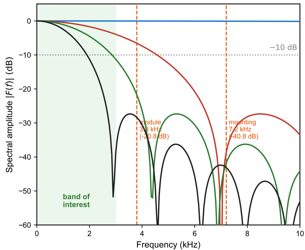
(d) Force spectra
