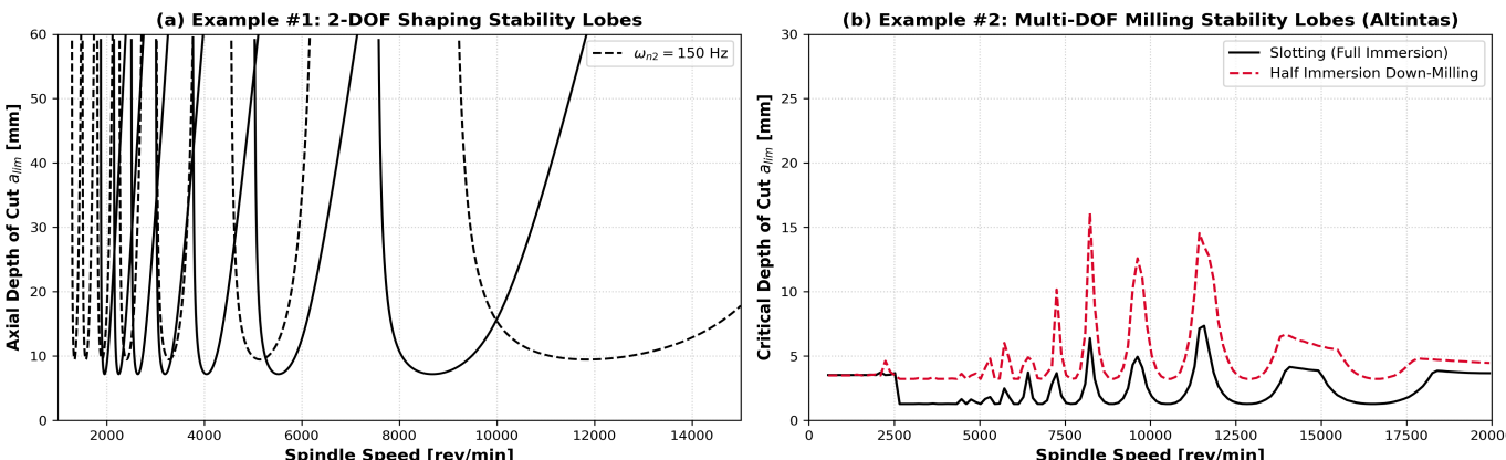
Hình 1: Tái lập giải tích Biểu đồ Búp Ổn định liên tục: (a) Máy bào 2 bậc tự do 2-DOF Shaping; (b) Phay rãnh Slotting & Phay biên Half-Immersion Down Milling (Altintas Example #1 & #2).
