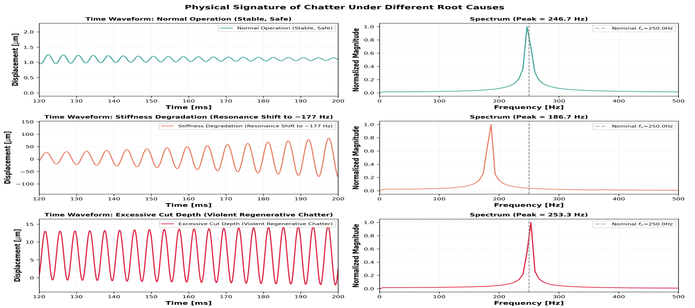
Hình 5: Dấu vân tay vật lý (Physical Signatures): Tín hiệu dịch chuyển theo thời gian và Phổ tần số FFT tương ứng với các dạng lỗi khác nhau.
