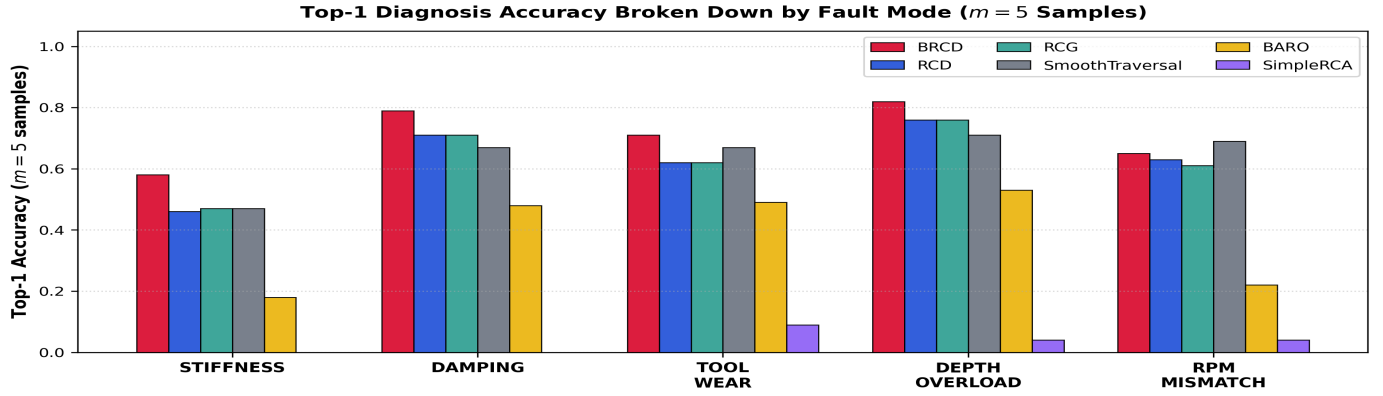
Hình 3: Biểu đồ cột phân tích Top-1 Accuracy theo từng kịch bản lỗi ở chế độ ít mẫu can thiệp ( m = 5 ).
