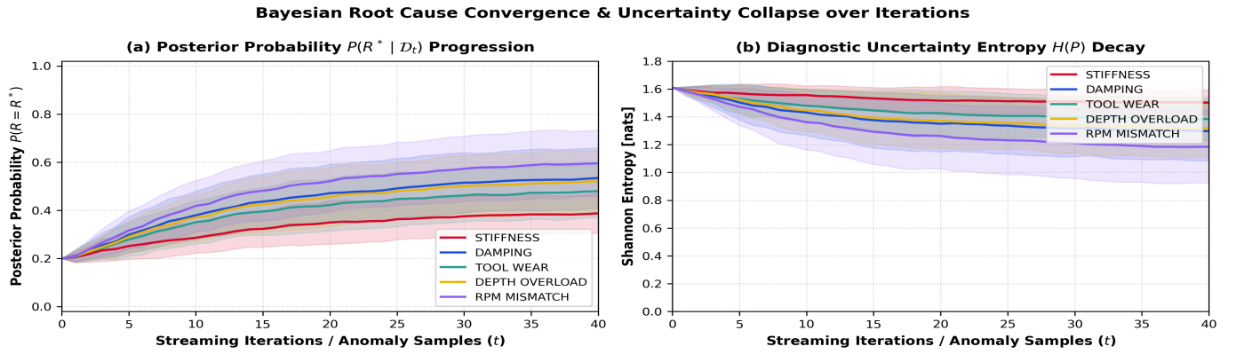
Hình 4: (a) Tiến trình tăng trưởng xác suất hậu nghiệm P(R^* \mid \mathcal{D}_t) ; (b) Đường suy giảm độ bất định Shannon H(P) qua 40 bước streaming.
