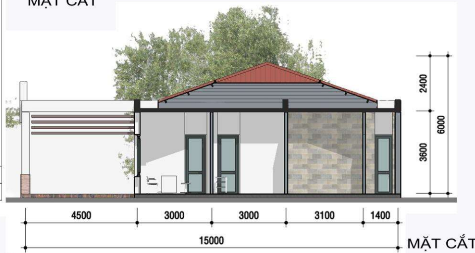
MẶT CẮT
