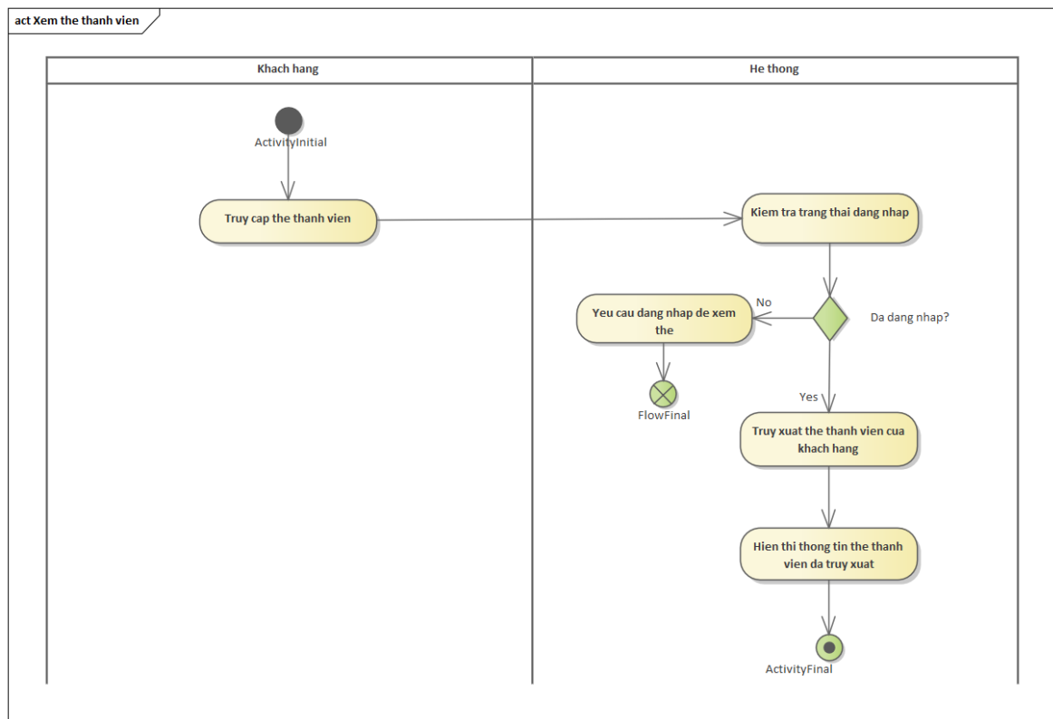
Hình 3.6: Sơ đồ hoạt động use case "Xem thẻ thành viên"
