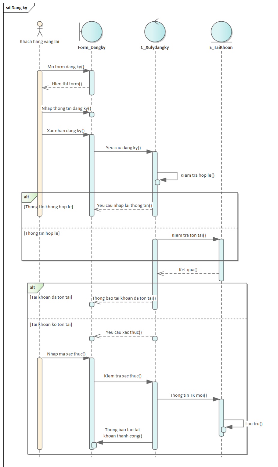
Hình 3.19: Sơ đồ tuần tự use case "Đăng ký"
