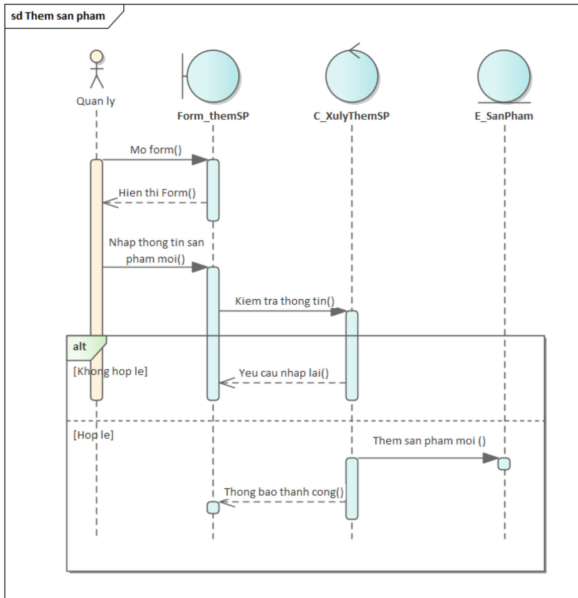
Hình 3.28: Sơ đồ tuần tự use case "Thêm sản phẩm"
