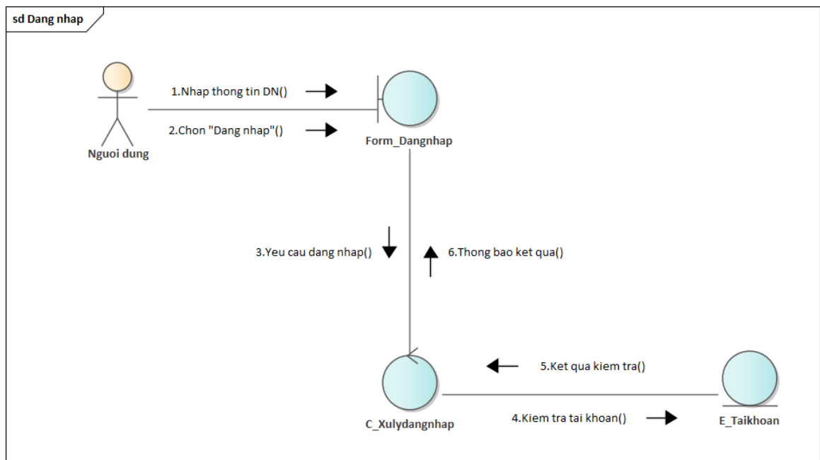
Hình 3.39: Sơ đồ cộng tác use case "Đăng nhập"
