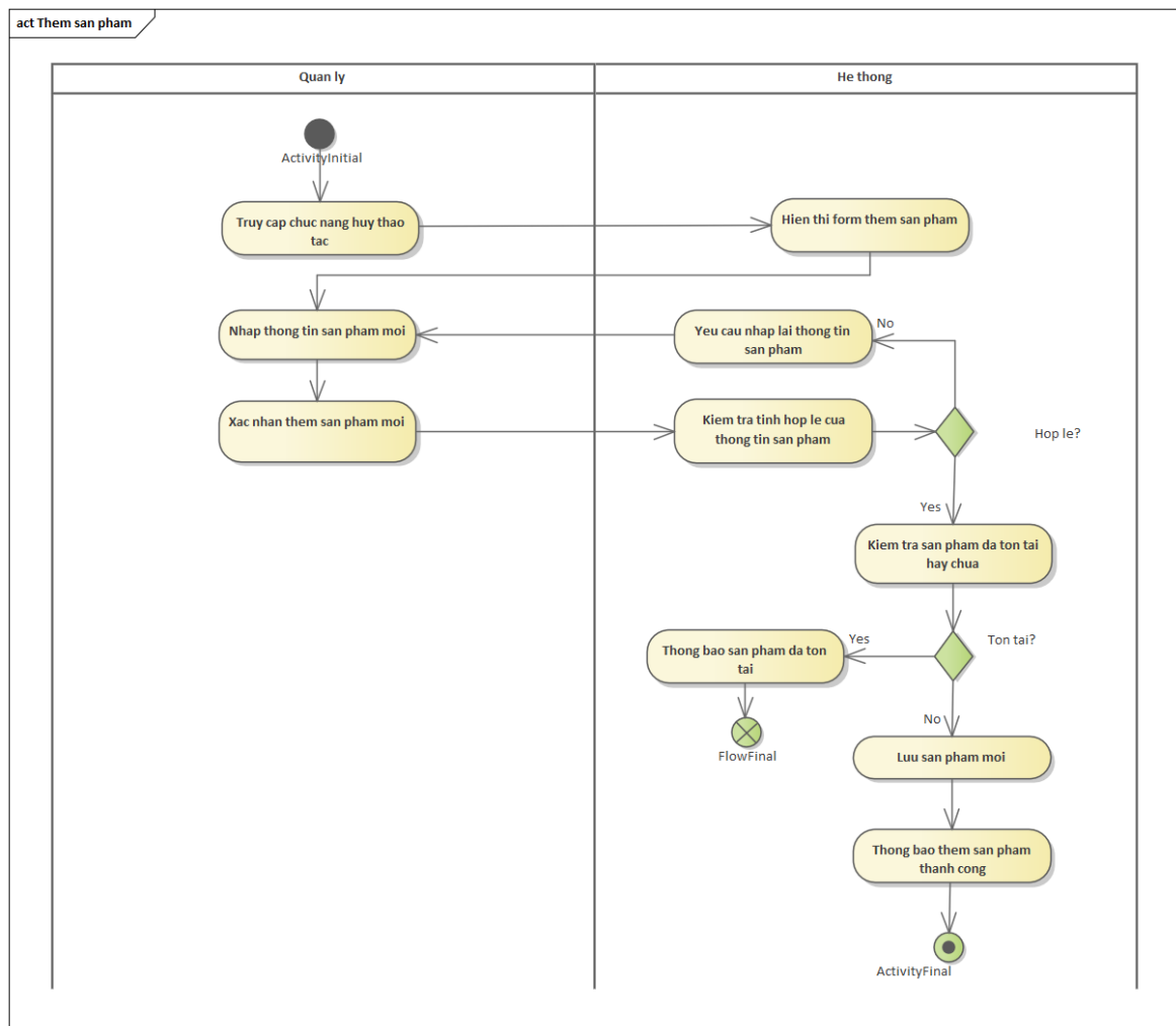
Hình 3.14: Sơ đồ hoạt động use case "Thêm sản phẩm"
