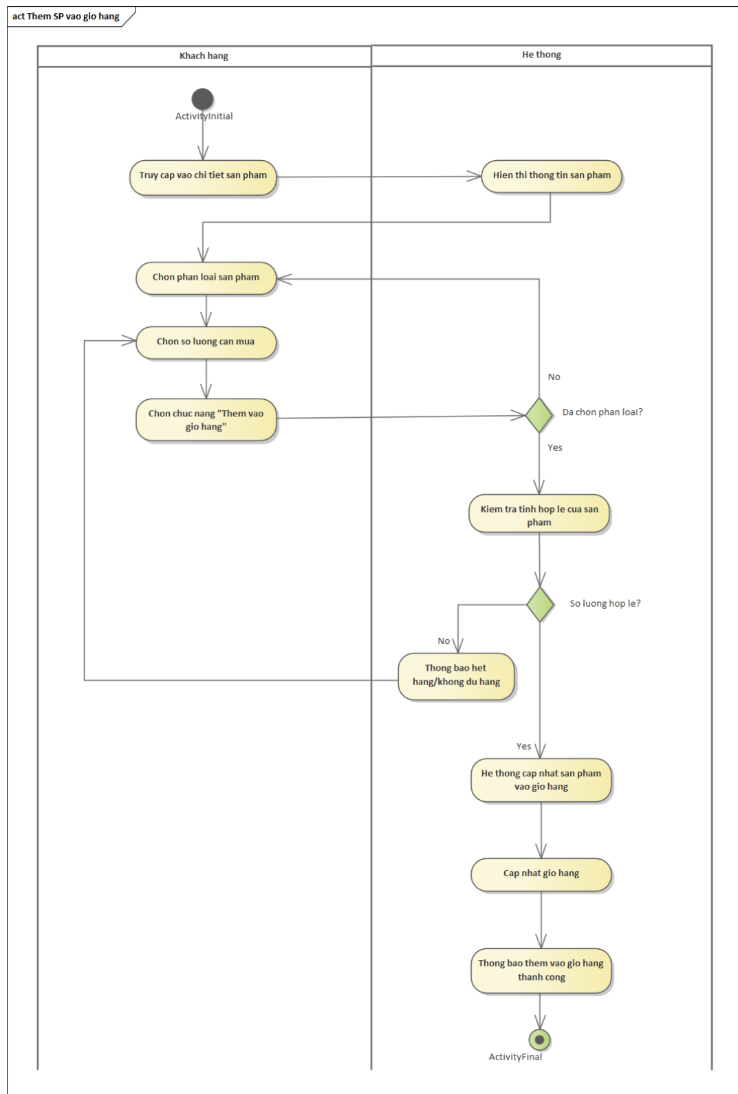
Hình 3.2: Sơ đồ hoạt động use case "Thêm sản phẩm vào giỏ hàng"
