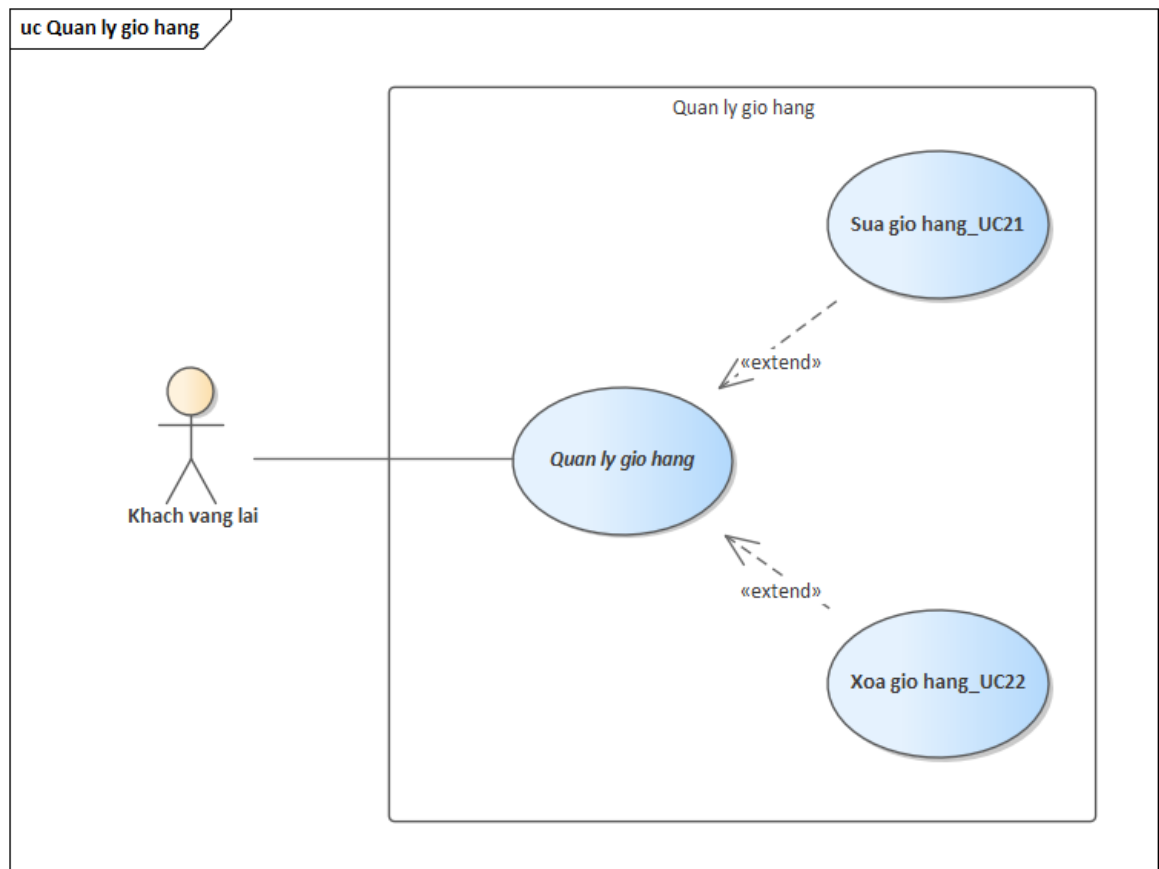
Hình 2.2: Sơ đồ use case chức năng quản lý giỏ hàng
