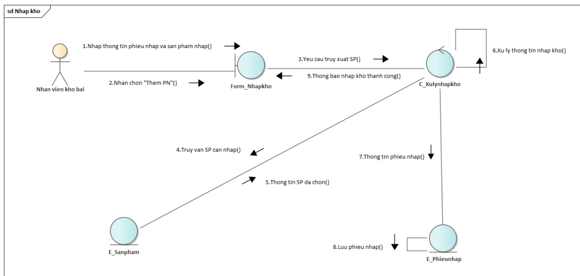
Hình 3.41: Sơ đồ cộng tác use case "Nhập kho"
