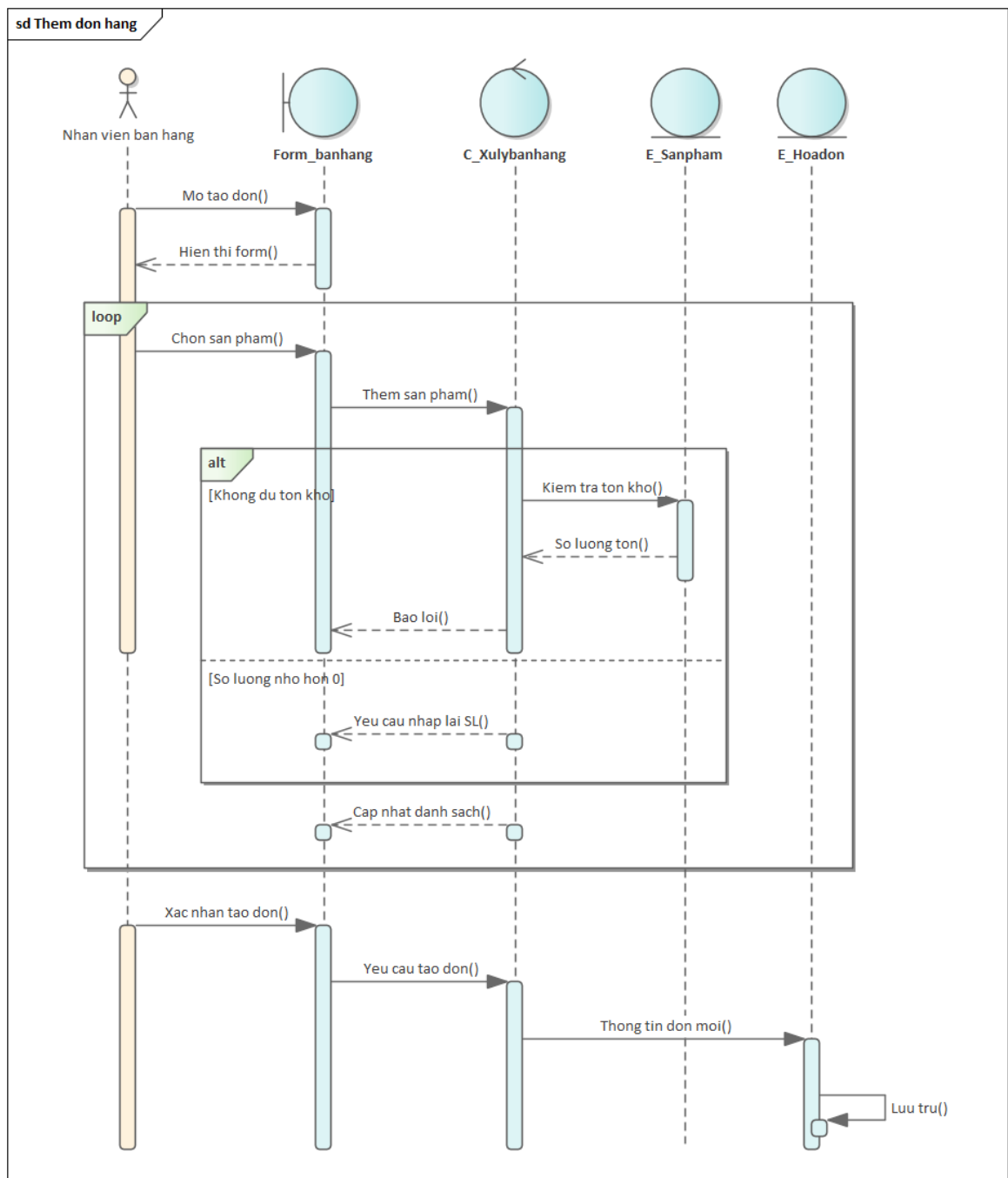
Hình 3.26: Sơ đồ tuần tự use case "Thêm đơn hàng"
