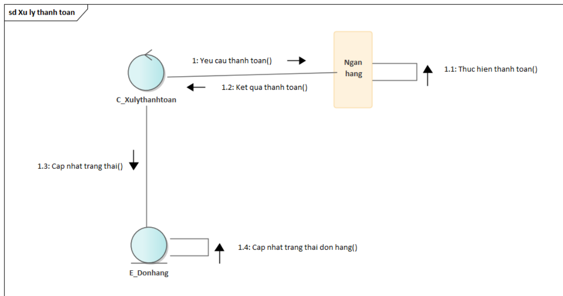
Hình 3.37: Sơ đồ cộng tác use case "Xử lý thanh toán"
