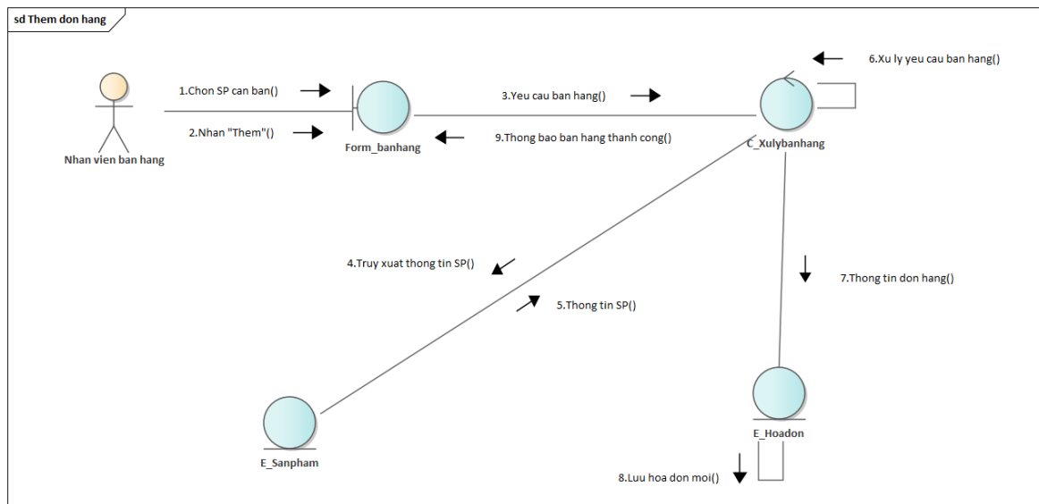
Hình 3.40: Sơ đồ cộng tác use case "Thêm đơn hàng"
