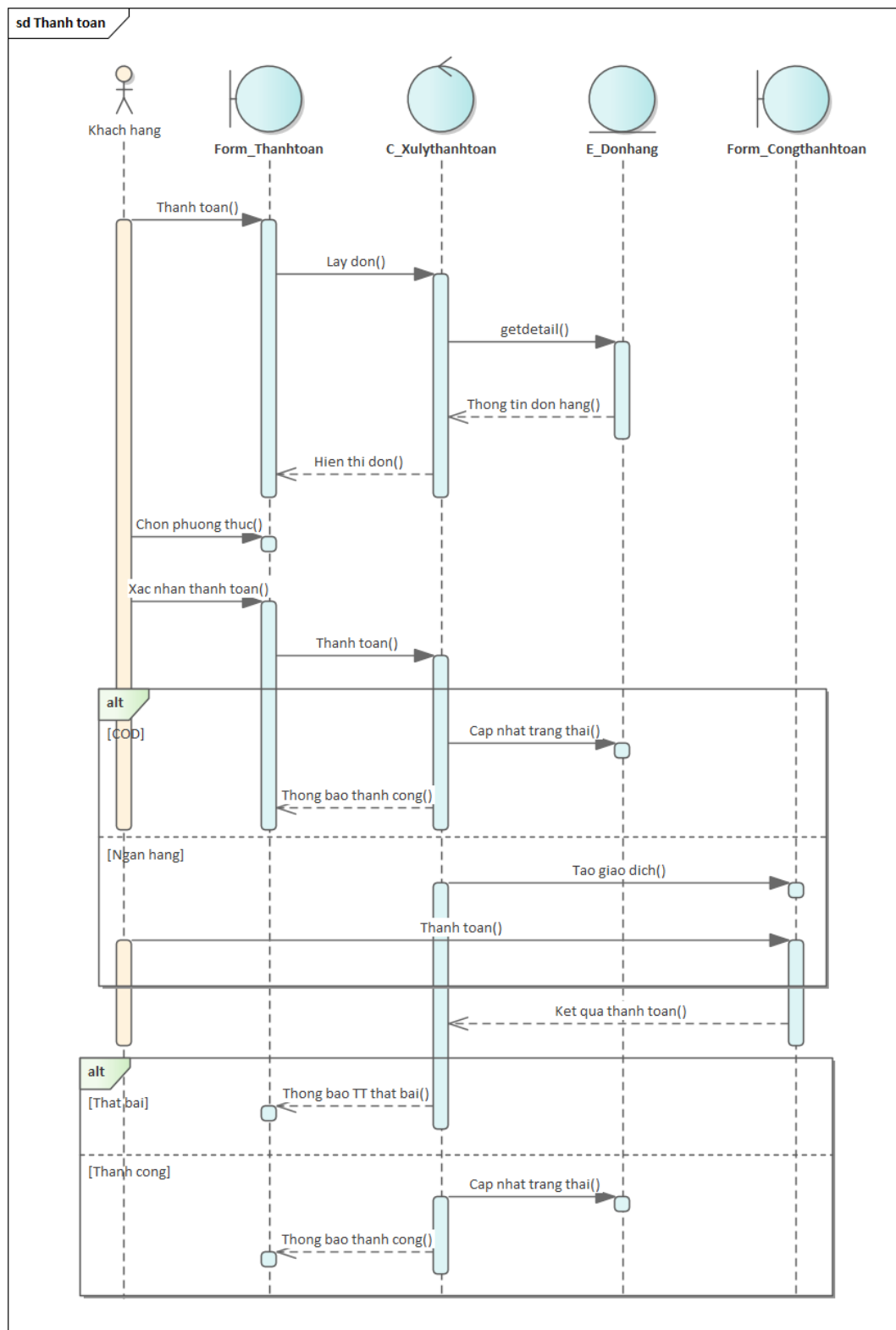
Hình 3.22: Sơ đồ tuần tự use case "Thanh toán"
