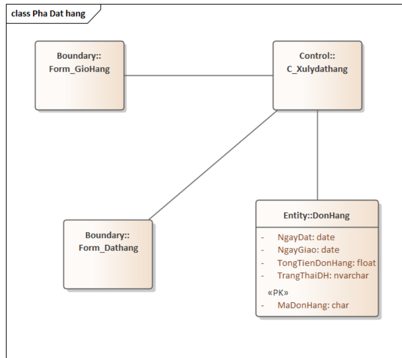
Hình 4.2: Pha đặt hàng
