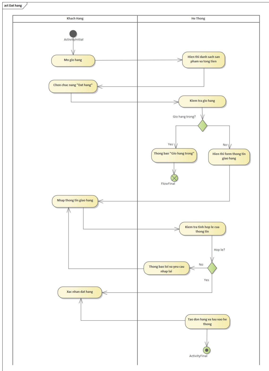
Hình 3.1: Sơ đồ hoạt động use case "Đặt hàng"
