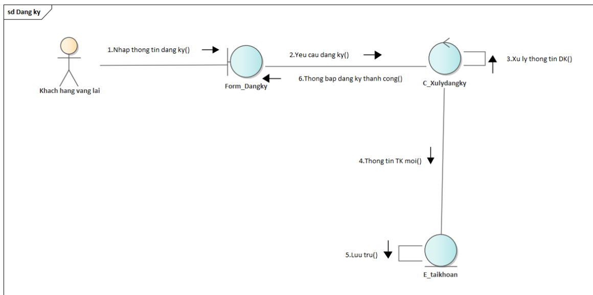
Hình 3.33: Sơ đồ cộng tác use case "Đăng ký"
