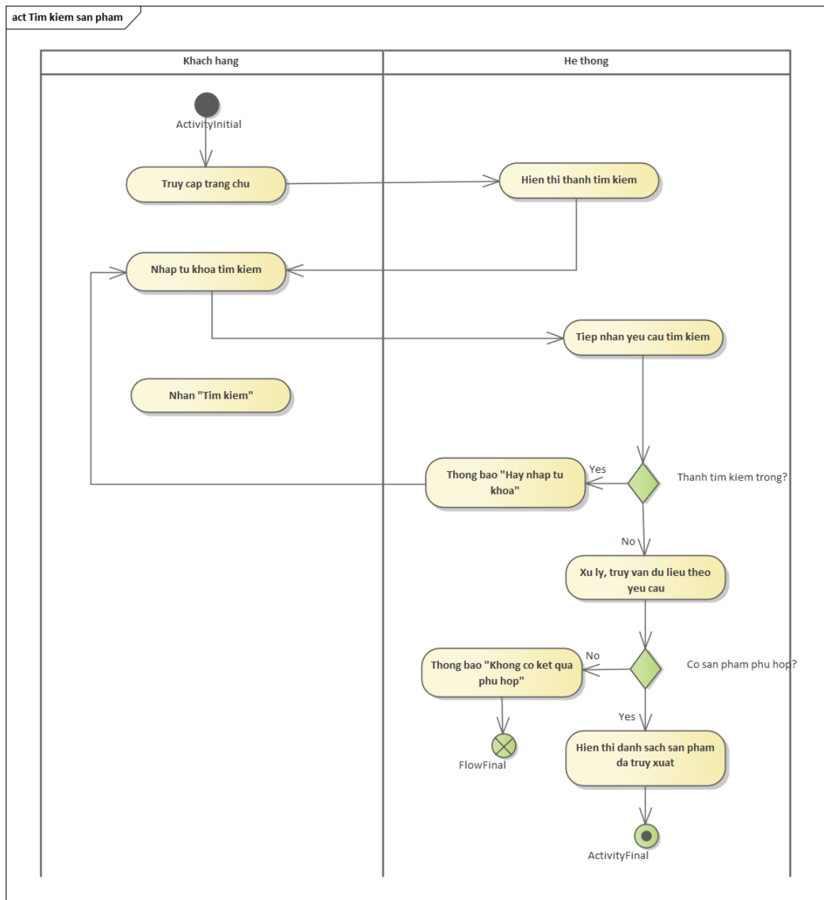
Hình 3.3: Sơ đồ hoạt động use case "Tìm kiếm sản phẩm"
