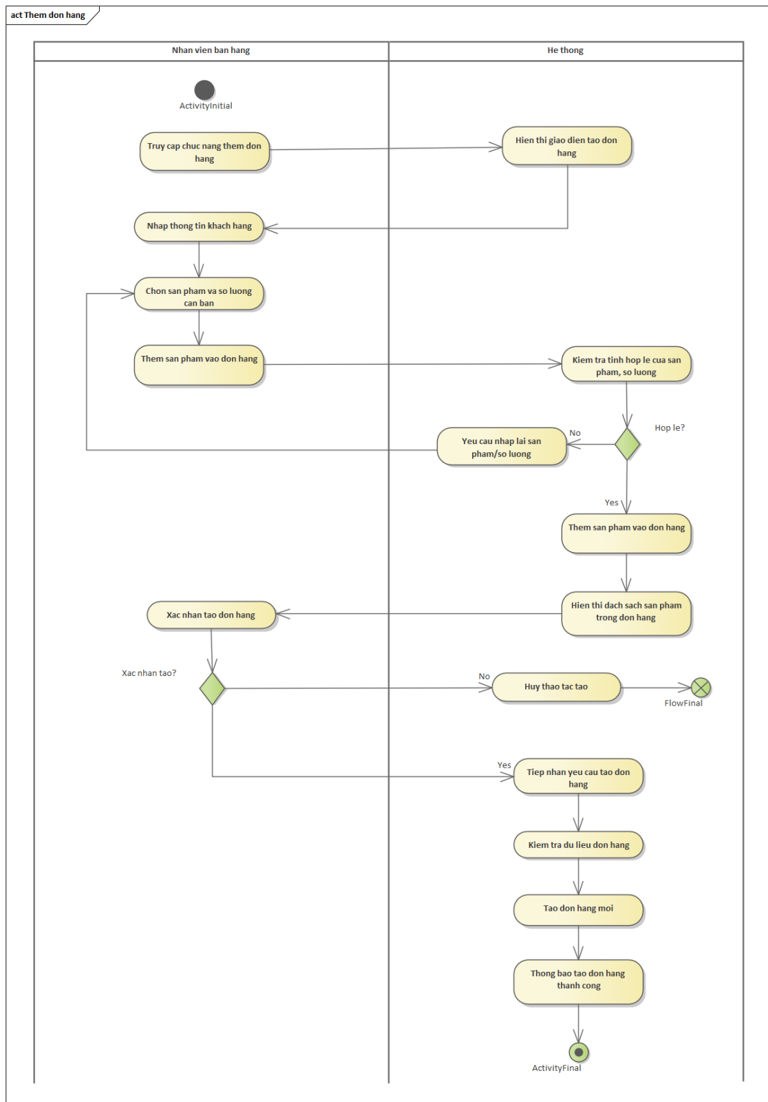
Hình 3.12: Sơ đồ hoạt động use case "Thêm đơn hàng"
