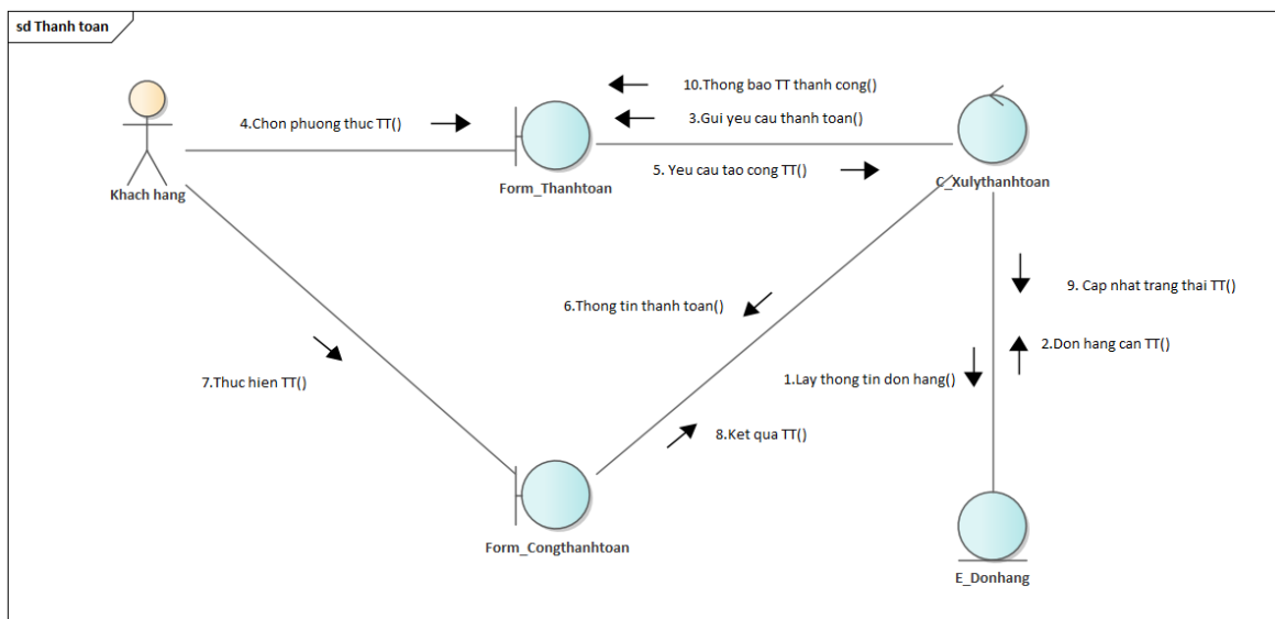
Hình 3.36: Sơ đồ cộng tác use case "Thanh toán"
