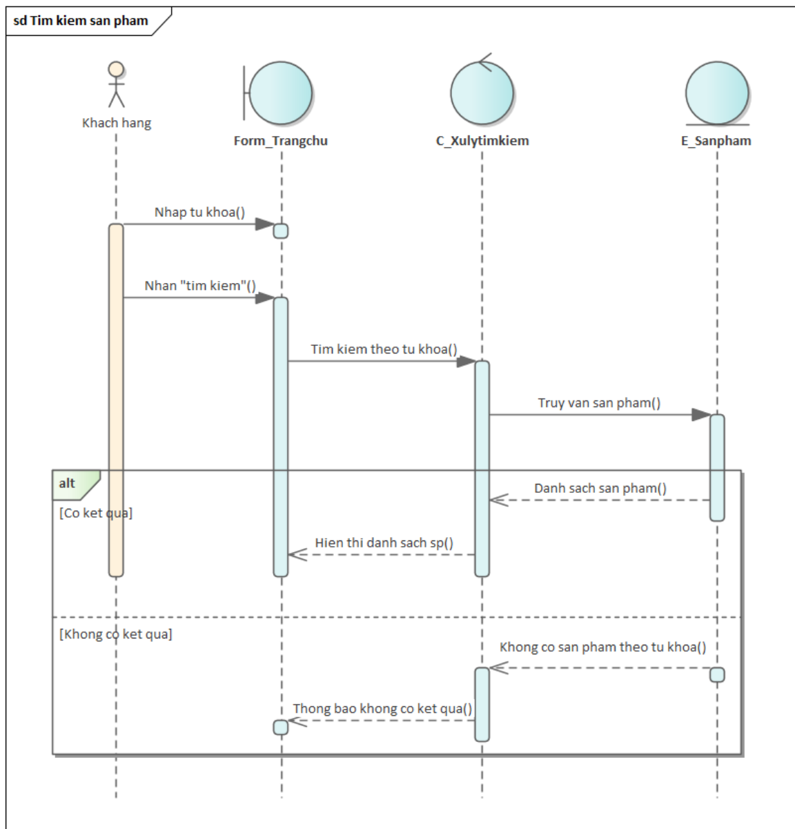
Hình 3.17: Sơ đồ tuần tự use case "Tìm kiếm sản phẩm"
