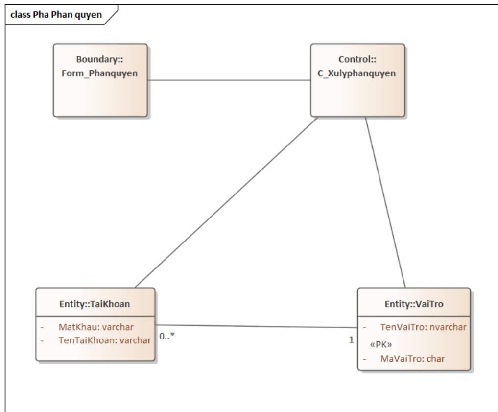
Hình 4.11: Pha phân quyền
