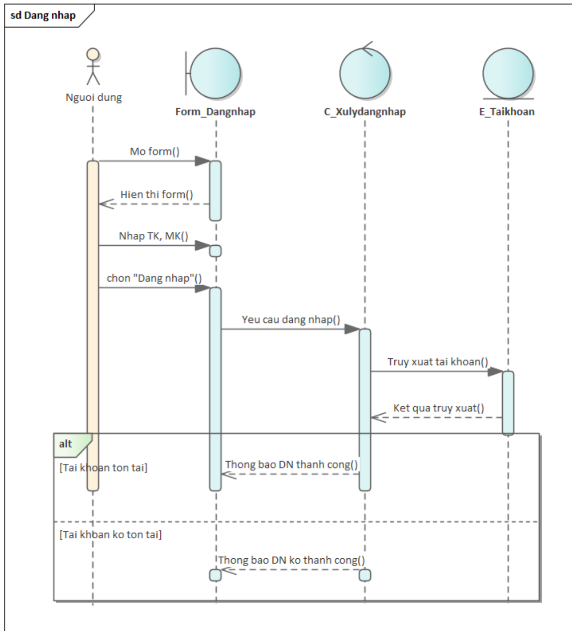
Hình 3.25: Sơ đồ tuần tự use case "Đăng nhập"
