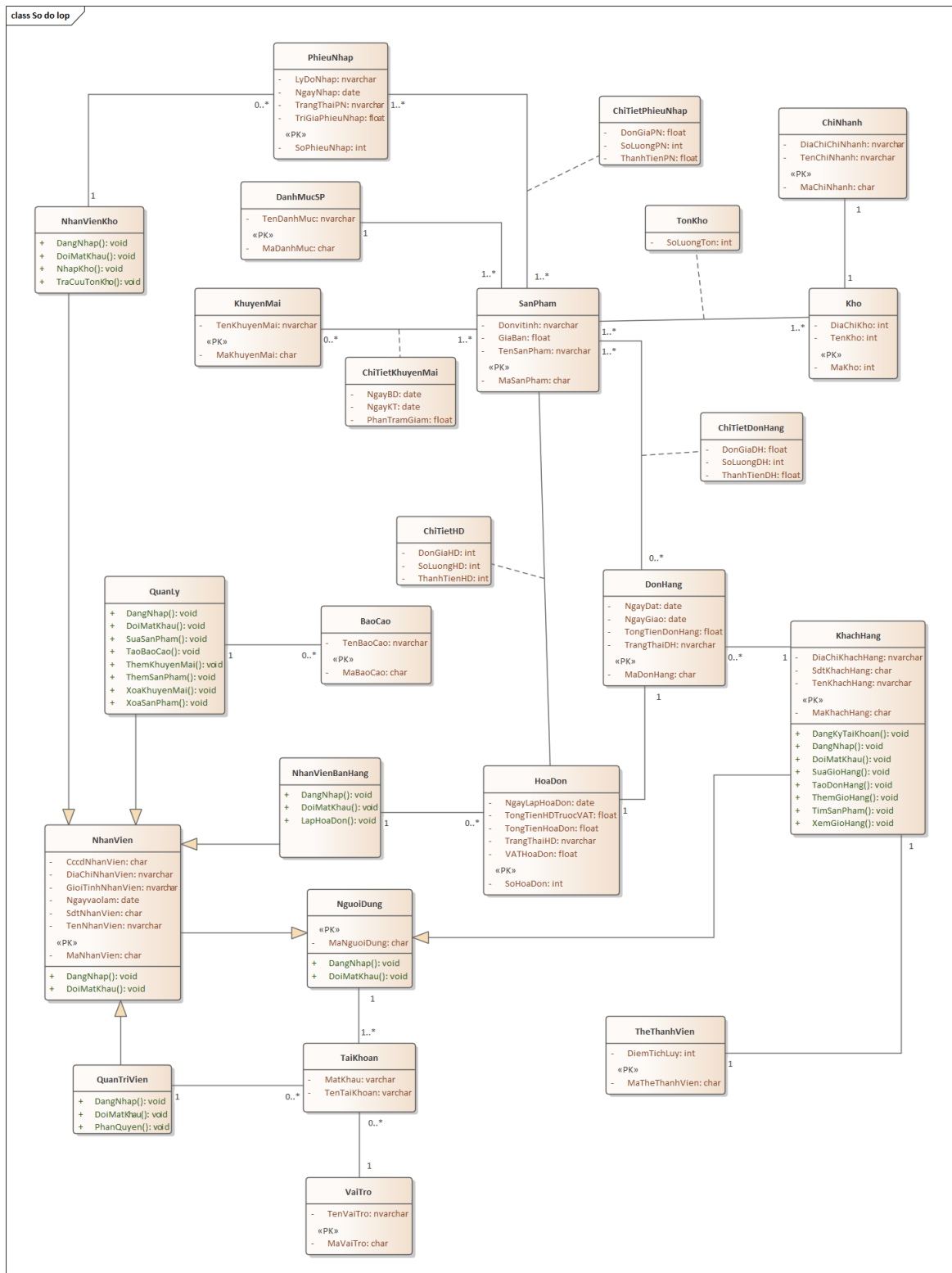
Hình 3.43: Sơ đồ Class hệ thống bán hàng online GS25
