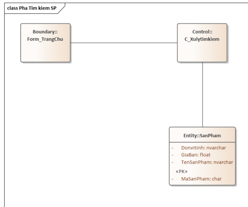
Hình 4.4: Pha tìm kiếm sản phẩm
