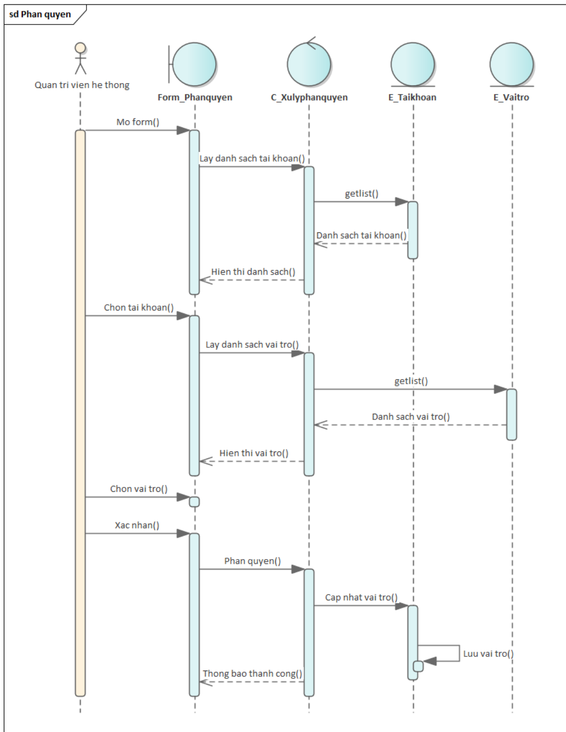
Hình 3.24: Sơ đồ tuần tự use case "Phân quyền"
