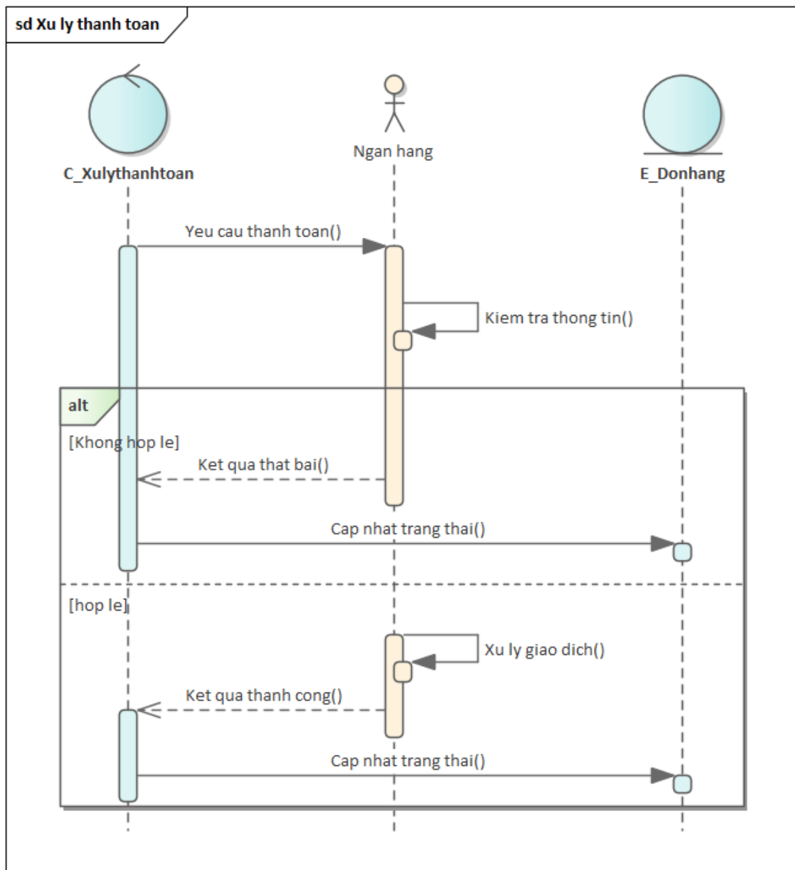
Hình 3.23: Sơ đồ tuần tự use case "Xử lý thanh toán"
