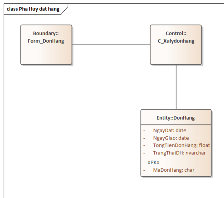
Hình 4.5: Pha hủy đặt hàng
