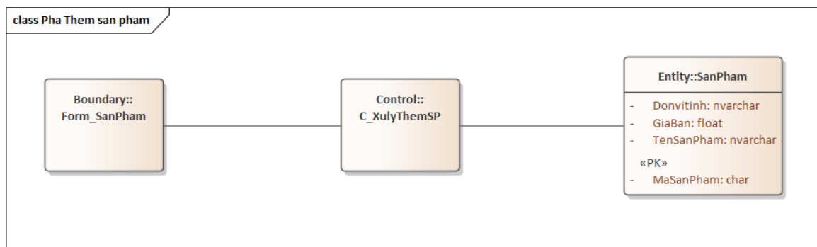
Hình 4.15: Pha thêm sản phẩm
