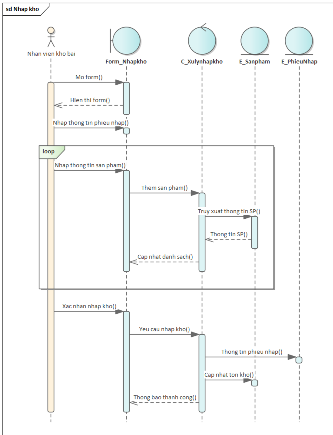
Hình 3.27: Sơ đồ tuần tự use case "Nhập kho"
