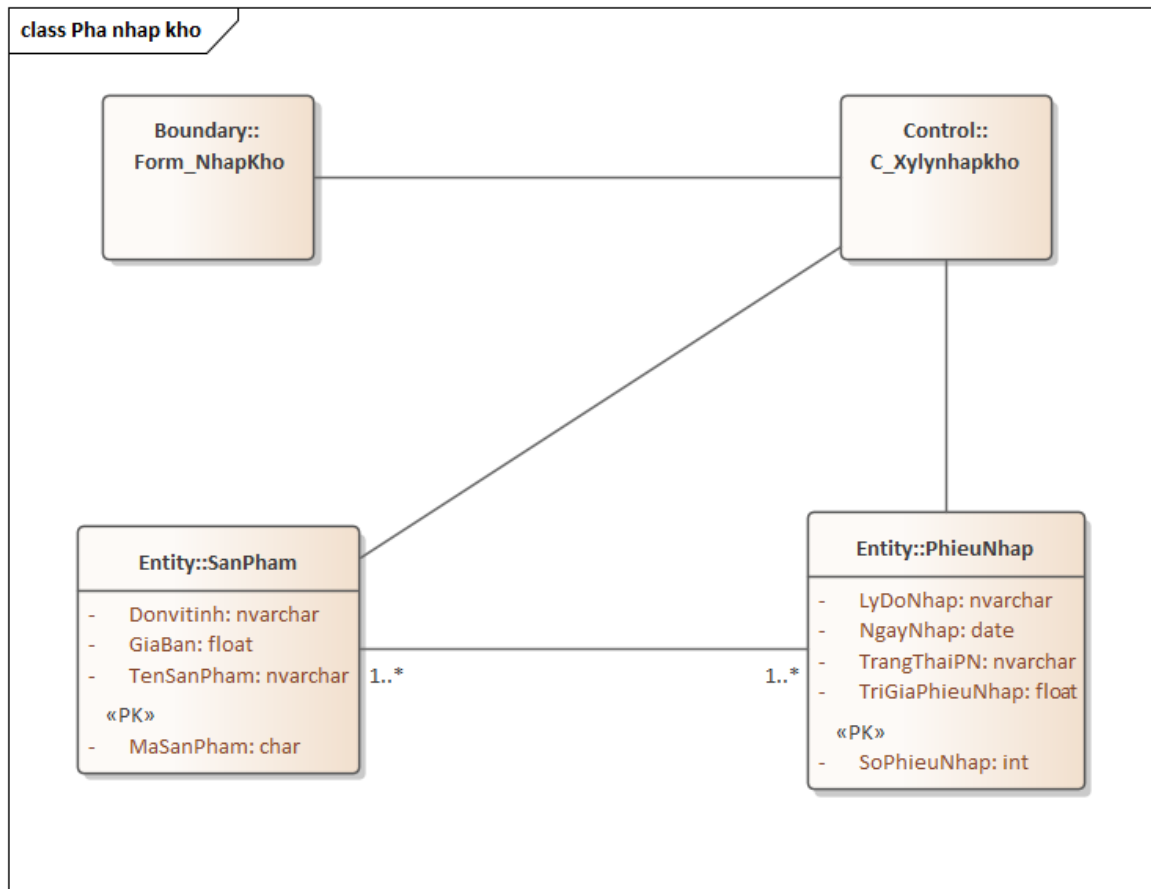
Hình 4.14: Pha nhập kho
