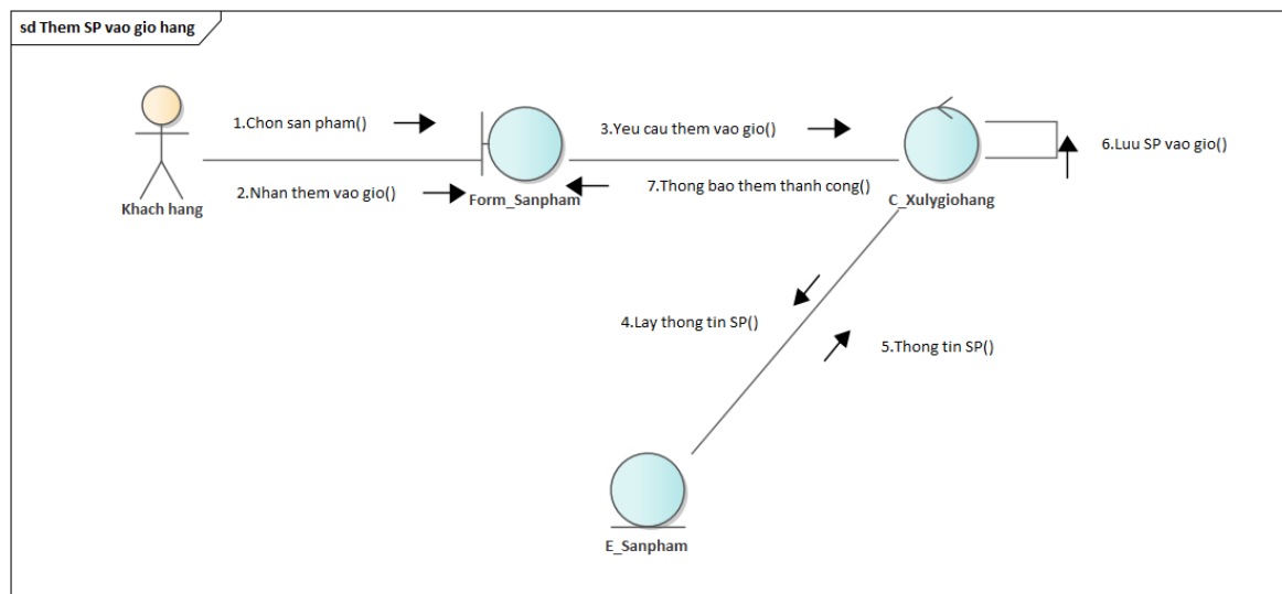
Hình 3.30: sơ đồ cộng tác use case "Thêm sản phẩm vào giỏ hàng"
