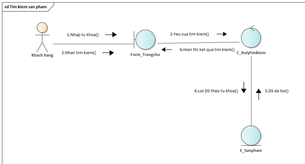
Hình 3.31: Sơ đồ cộng tác use case "Tìm kiếm sản phẩm"
