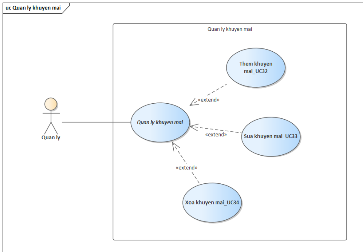
Hình 2.6: Sơ đồ use case chức năng quản lý khuyến mãi
