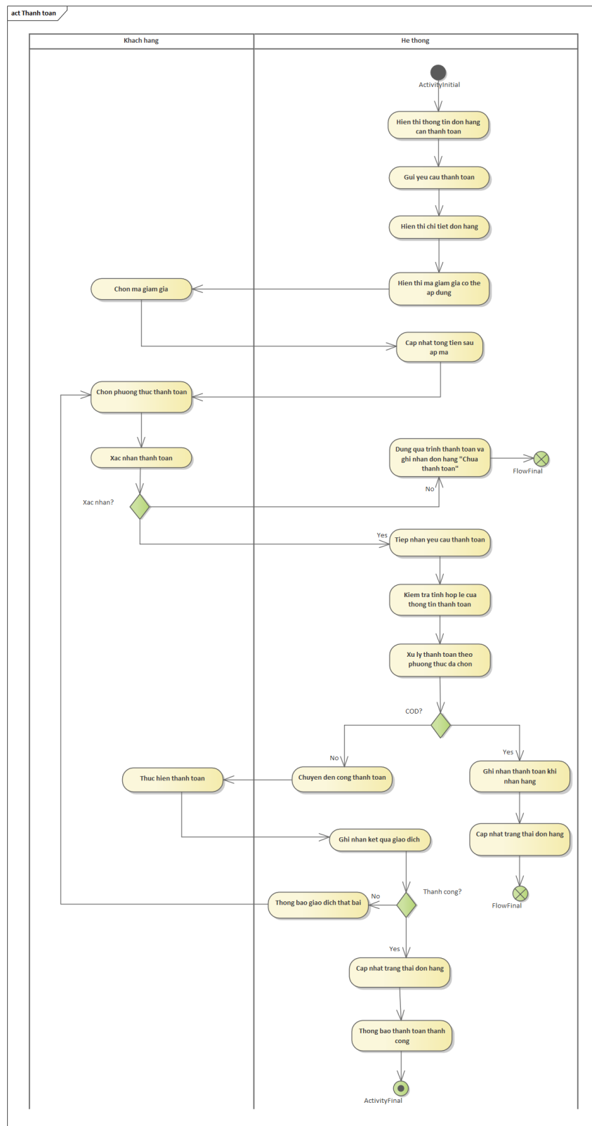
Hình 3.8: Sơ đồ hoạt động "Thanh toán"
