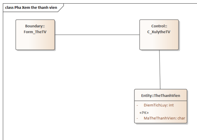
Hình 4.7: Pha xem thẻ thành viên
