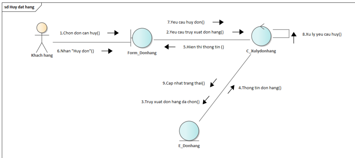
Hình 3.32: Sơ đồ cộng tác use case "Hủy đặt hàng"
