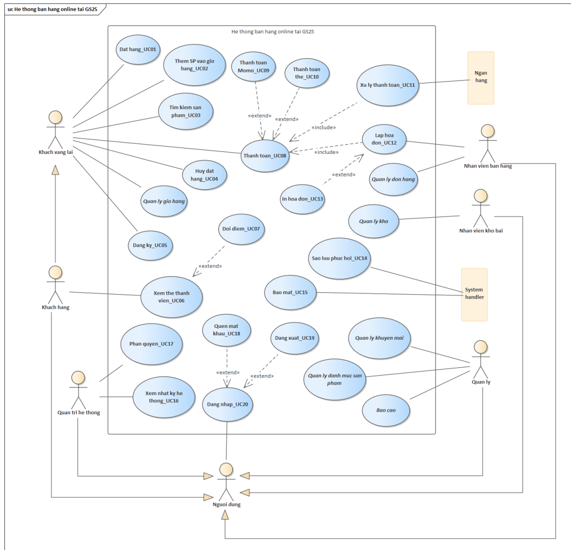
Hình 2.1: Sơ đồ use case mức tổng thể
