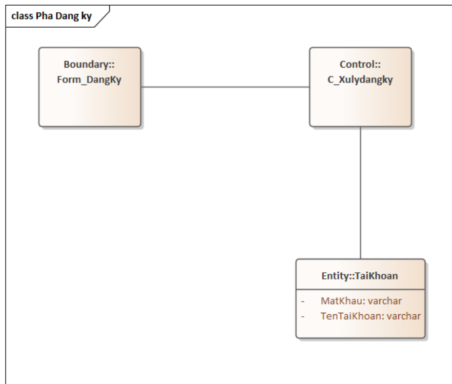
Hình 4.6: Pha đăng ký
