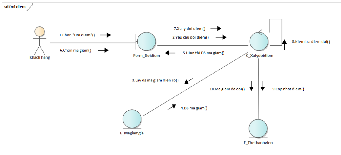
Hình 3.35: Sơ đồ cộng tác use case "Đổi điểm"
