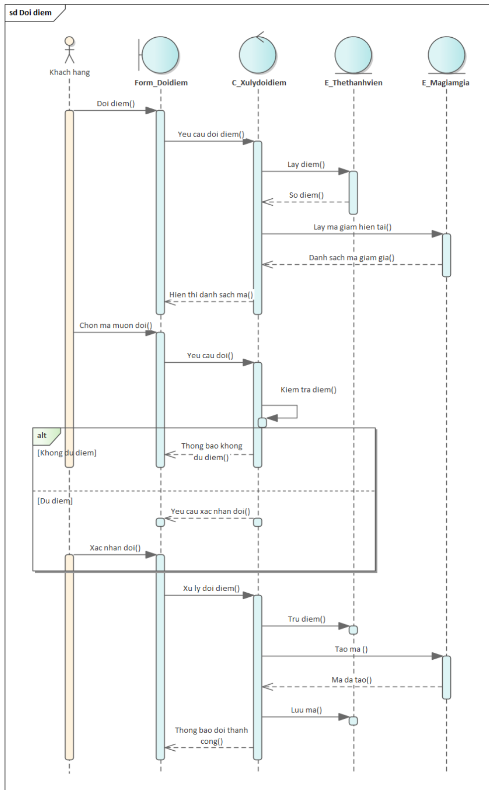
Hình 3.21: Sơ đồ tuần tự use case "Đổi điểm"
