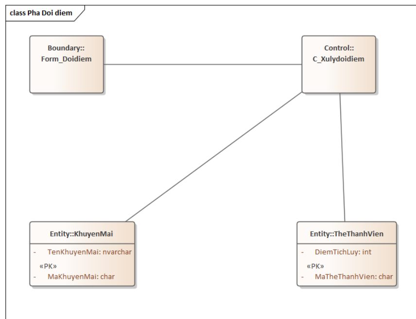
Hình 4.8: Pha đổi điểm
