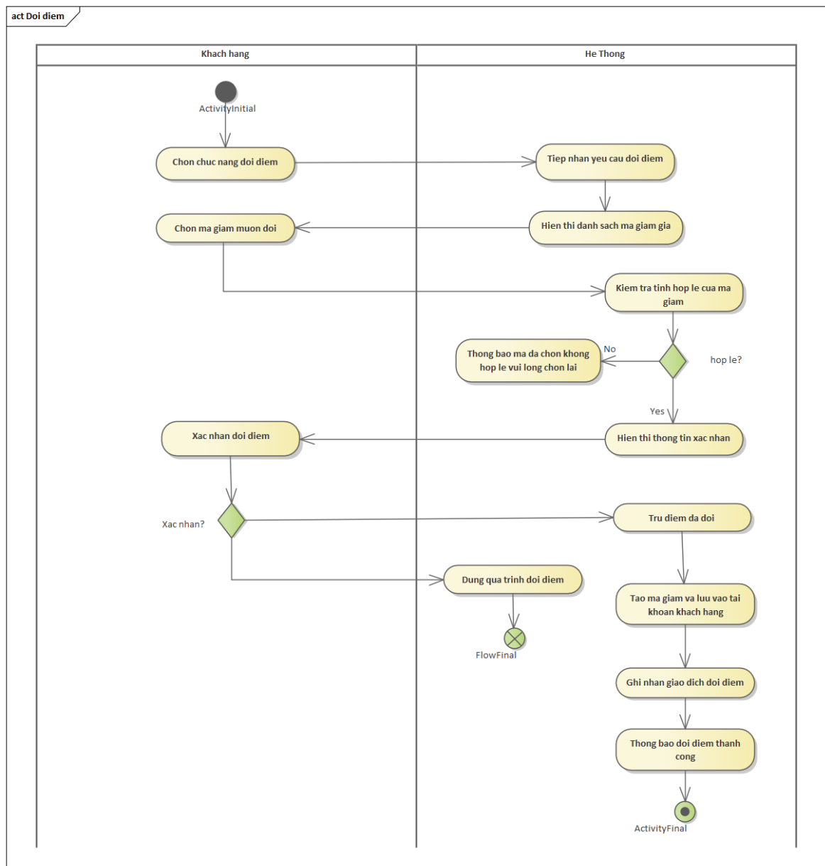
Hình 3.7: Sơ đồ hoạt động use case "Đổi điểm"
