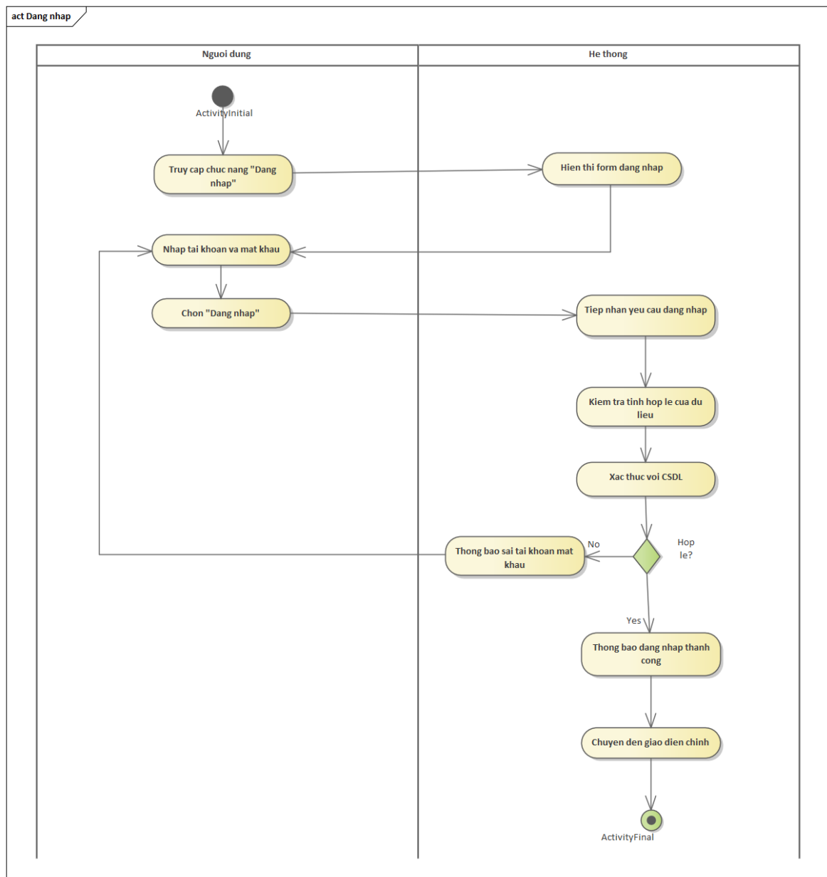
Hình 3.11: Sơ đồ hoạt động use case "Đăng nhập"
