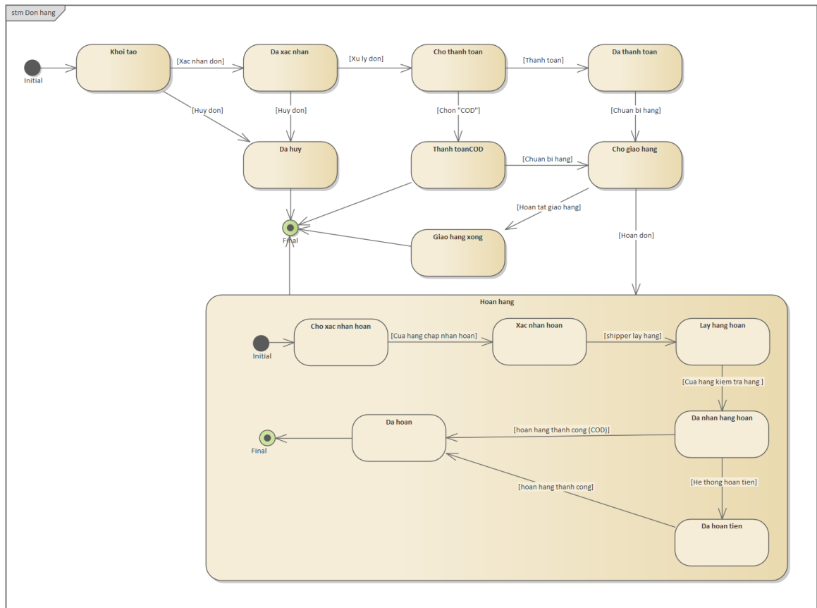
Hình 3.44: Sơ đồ trạng thái lớp "Đơn hàng"
