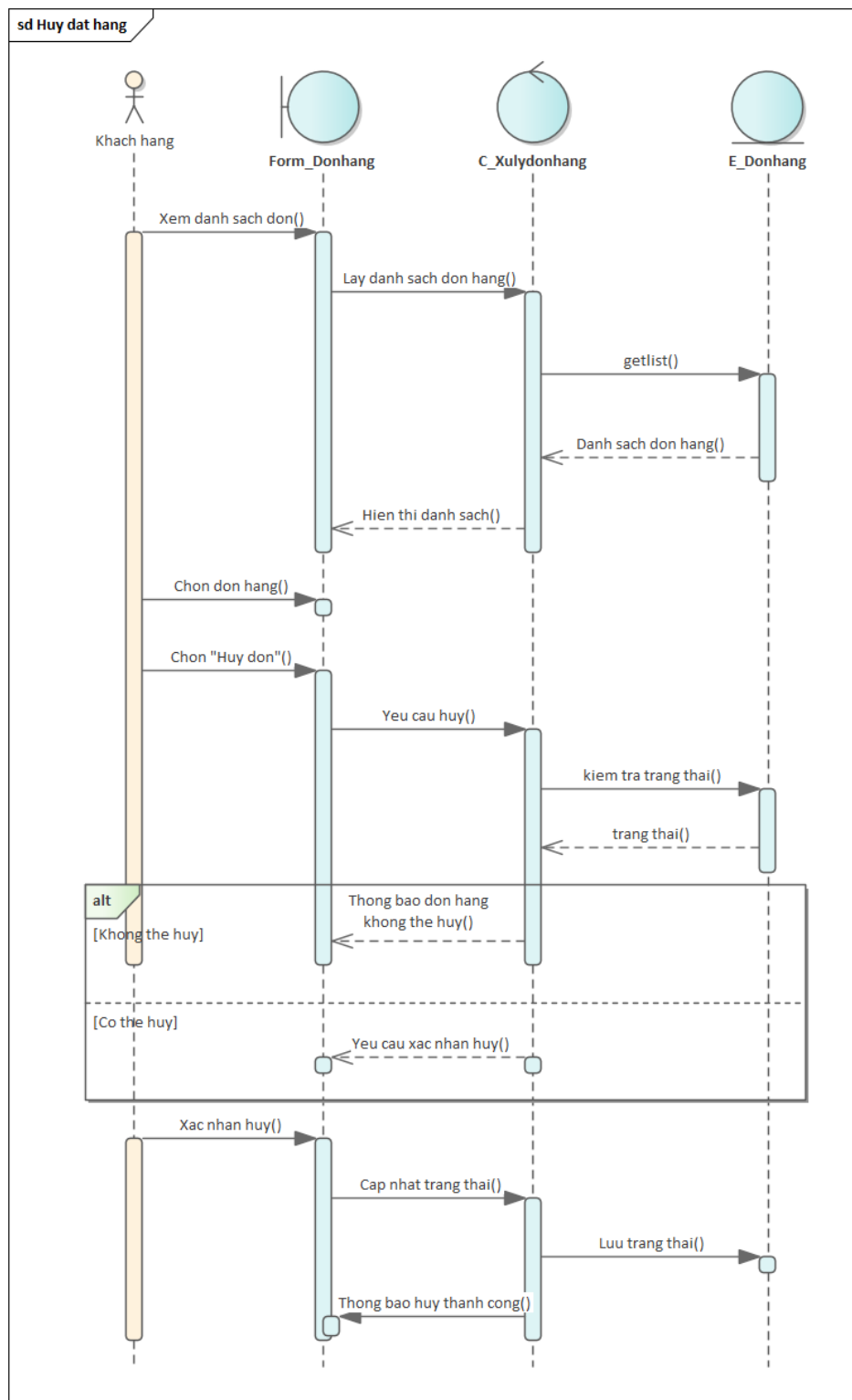
Hình 3.18: Sơ đồ tuần tự use case "Hủy đặt hàng"
