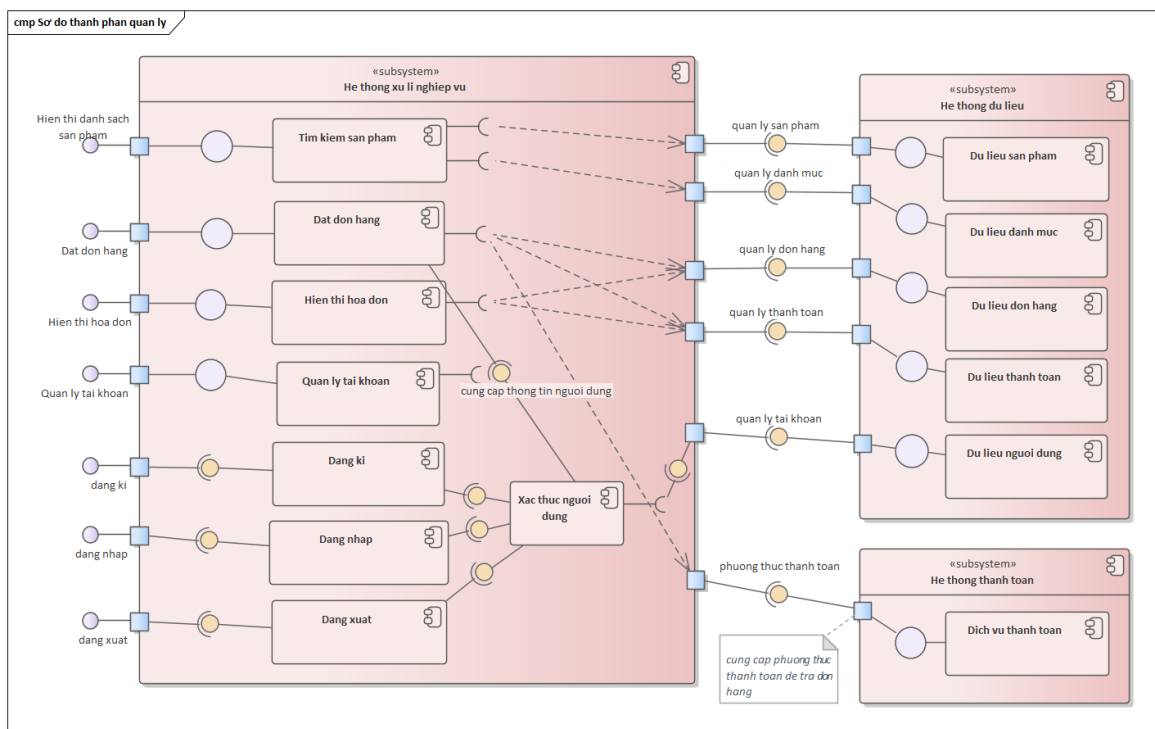
Hình 4.71: sơ đồ thành phần quản lý
