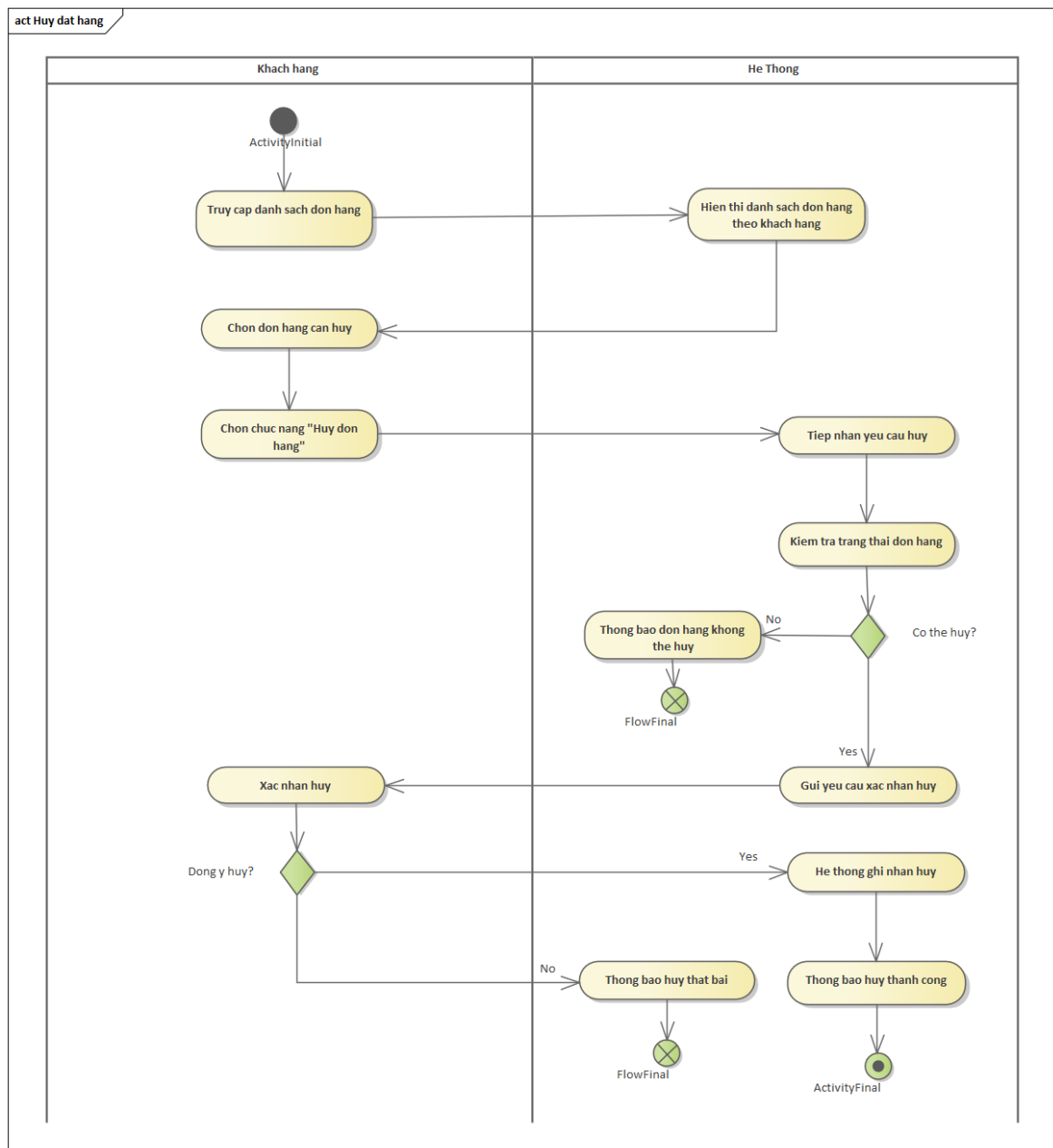
Hình 3.4: Sơ đồ hoạt động use case "Hủy đặt hàng"
