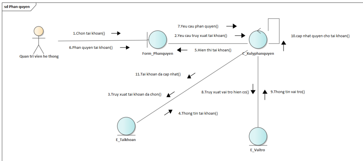
Hình 3.38: Sơ đồ cộng tác use case "Phân quyền"
