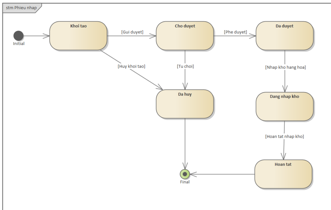
Hình 3.46: Sơ đồ trạng thái lớp "Phiếu nhập"
