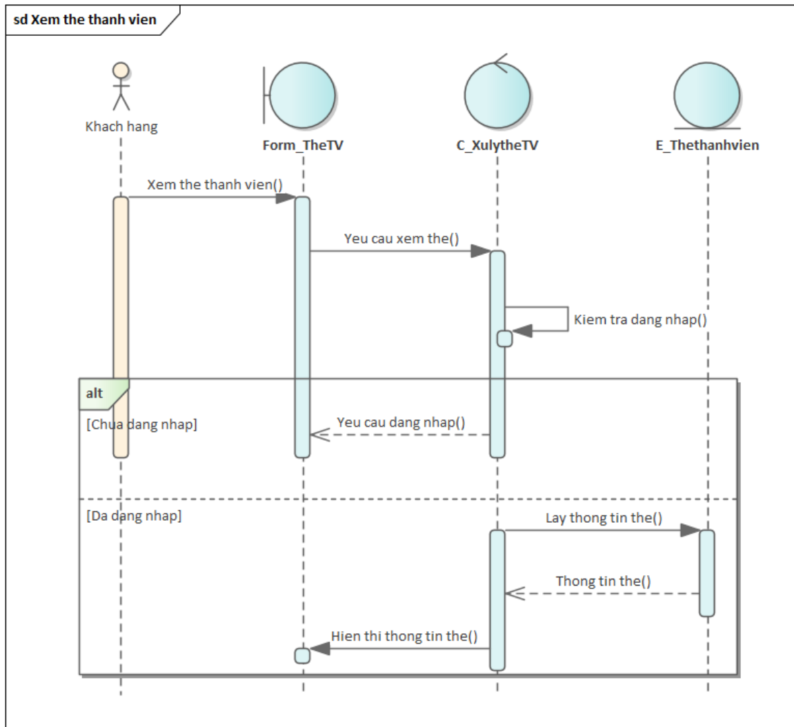
Hình 3.20: Sơ đồ tuần tự use case "Xem thẻ thành viên"
