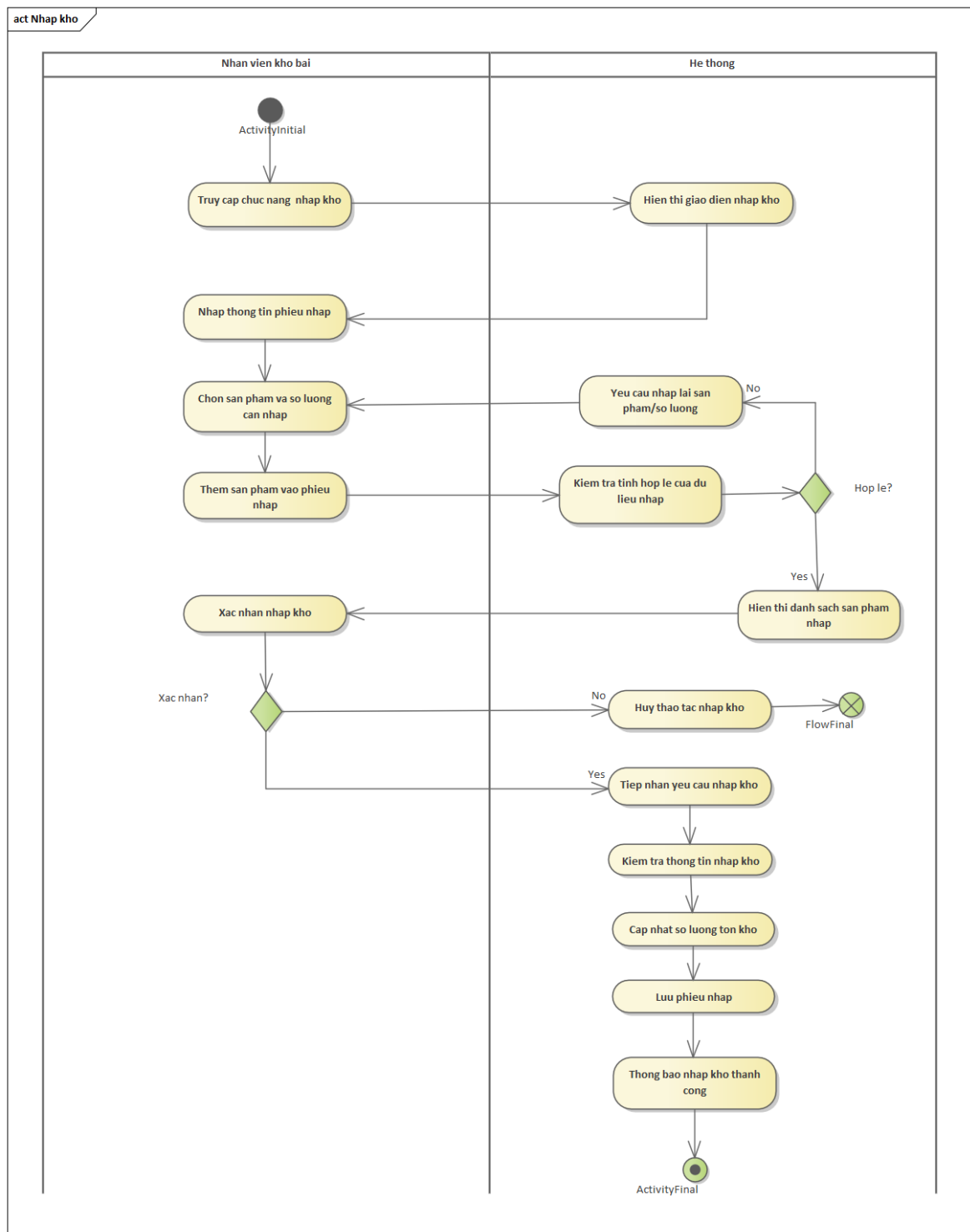
Hình 3.13: Sơ đồ hoạt động use case "Nhập kho"
