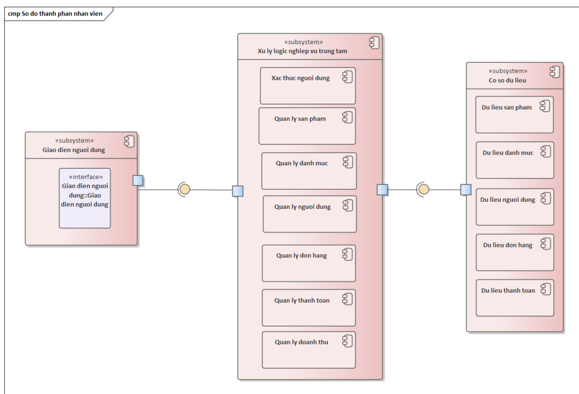
Hình 4.70: Sơ đồ thành phần nhân viên
