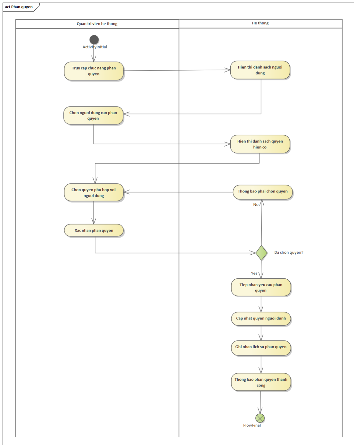
Hình 3.10: Sơ đồ hoạt động use case "Phân quyền"
