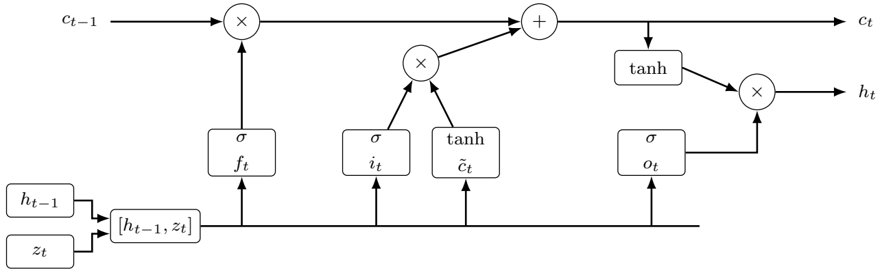
Рис. 1 – Блок-схема LSTM-ячейки
