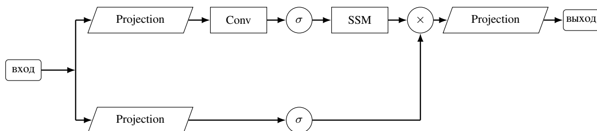
Рис. 4 – Блок-схема Mamba-блока
