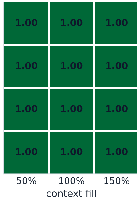
GPT-4o-mini
