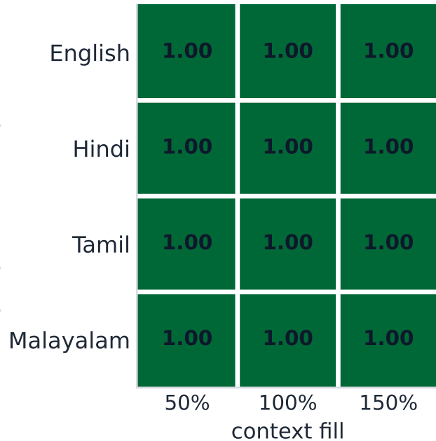
Llama-3.1-8B
