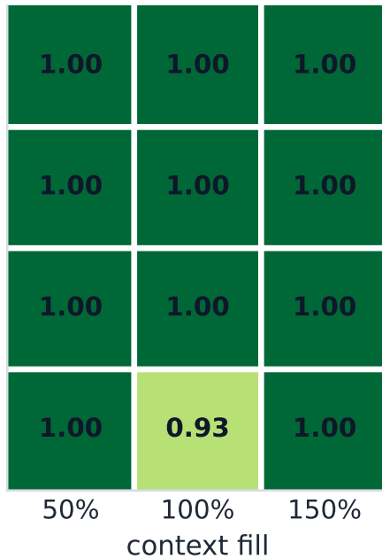
GPT-3.5-Turbo
