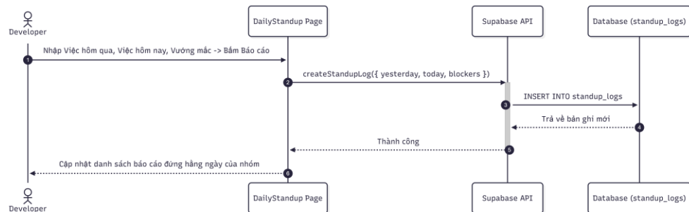
Hình 3.10: Sơ đồ tuần tự cho chức năng Tạo nhật ký Daily Standup
