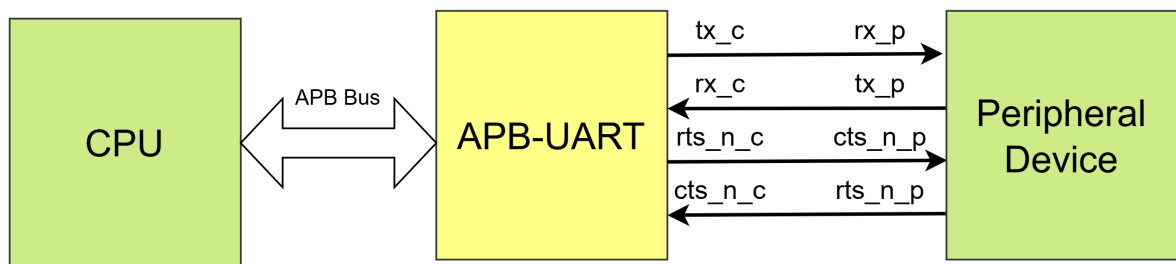
Hình 2: Hệ thống sử dụng apb_uart
