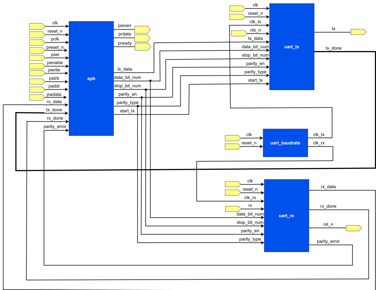
Hình 5: uart_apb architecture
