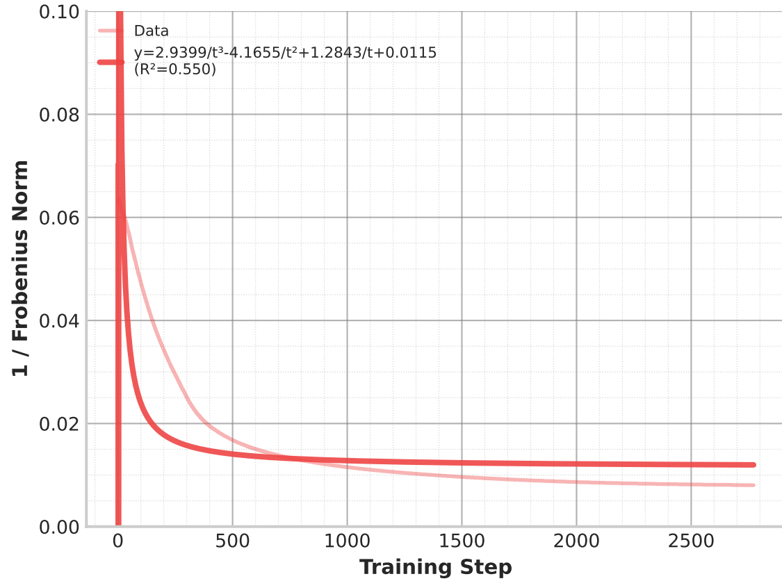
Block 0 - MLP Proj
