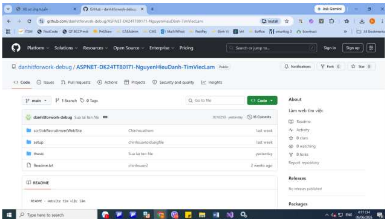
Hình 1 Github
