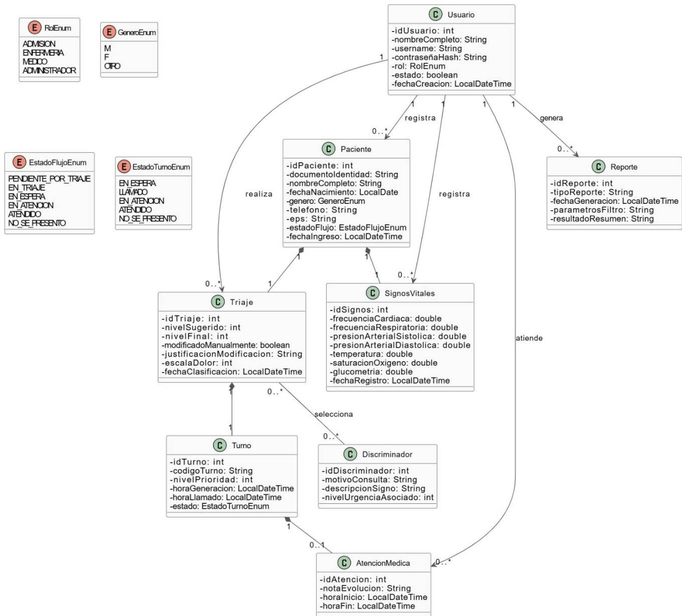
Figura 2 Diagrama UML
