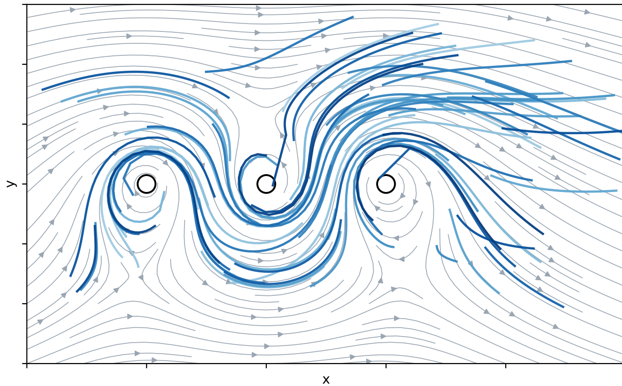
Dataset 1 (constant)
