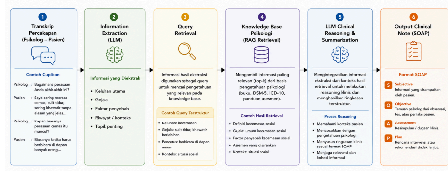
Gambar 2.3 Posisi Information Extraction dalam Alur Sistem
