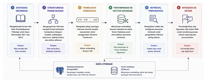
Gambar 3.2 Pipeline Pembangunan Knowledge Base Psikologi
