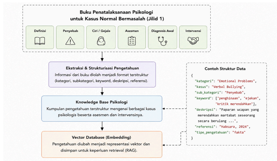
Gambar 2.2 Representasi Pengetahuan Psikologi untuk Sistem AI (Diadaptasi dari Habsara, 2024 [16])
