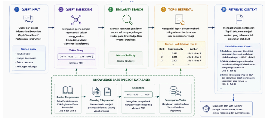
Gambar 3.3 Alur Modul RAG dari Query hingga Retrieved Context
