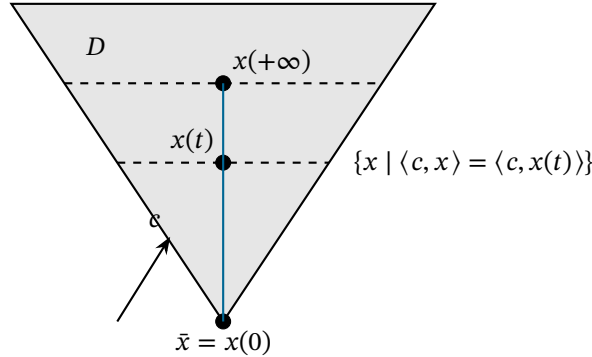
Figura 10.5.: El punto x(t) de la trayectoria central es el centro analítico de la intersección de D con el hiperplano donde el valor de la función objetivo es \langle c, x(t) \rangle .
