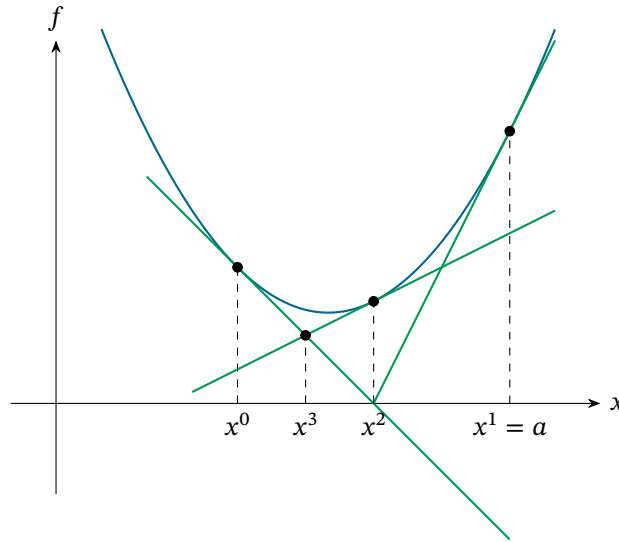
Figura 9.2.: Tres iteraciones del método de planos cortantes para la función f en el conjunto D = [0, a] . Se tiene que x^{k+1} es el minimizador de la aproximación \psi_k en D . Después de cada iteración, un plano cortante más es introducido en la aproximación: \psi_{k+1}(x) = \max\{\psi_k(x), f(x^{k+1}) + \langle y^{k+1}, x - x^{k+1} \rangle\} , y^{k+1} \in \partial f(x^{k+1}) .
