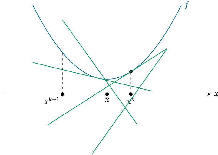
Figura 9.3.: La iteración del método de planos cortantes puede generar x^{k+1} para el cual la distancia a la solución y el valor de la función objetivo aumentan en comparación con el iterado anterior x^k .
