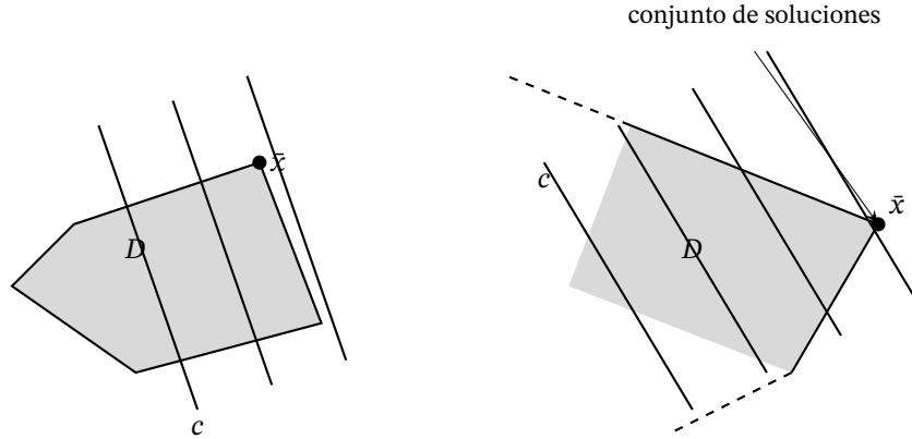
Figura 10.2.: Cuando un problema de programación lineal posee soluciones y el conjunto viable tiene vértices, uno de los vértices es solución del problema (en el dibujo, las rectas paralelas son curvas de nivel de la función objetivo \langle c, x \rangle ).
