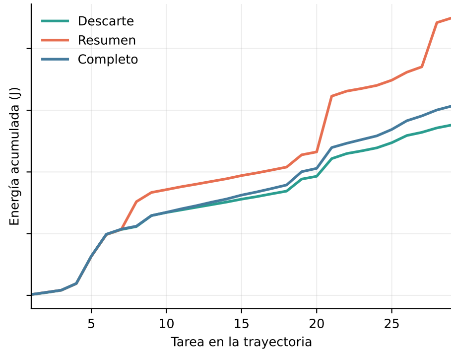
FP16
