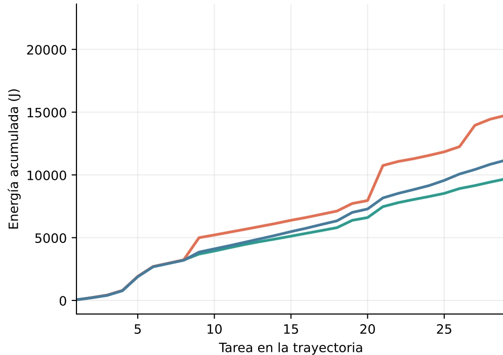
AWQ
