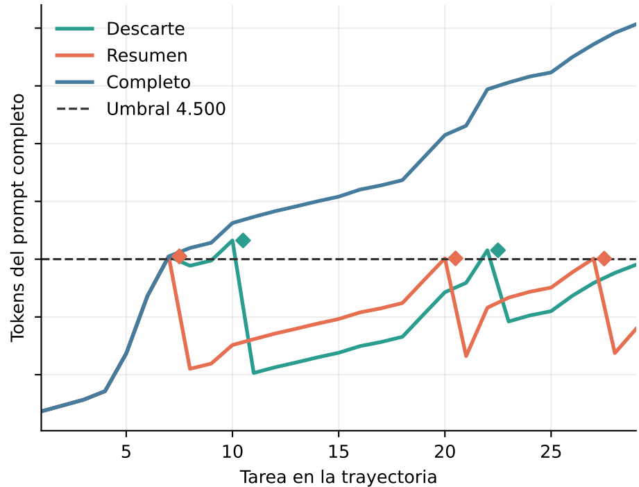
FP16
