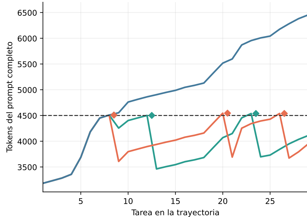
AWQ
