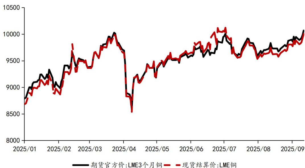
图 23：LME 铜价走势（美元/吨）
