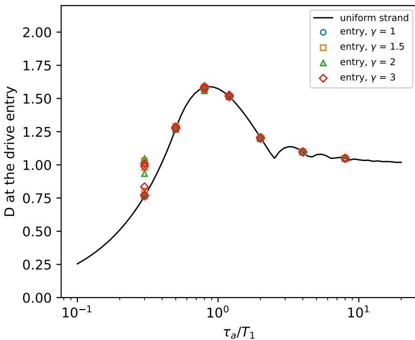
(d) loop, drive entry (all \xi )
