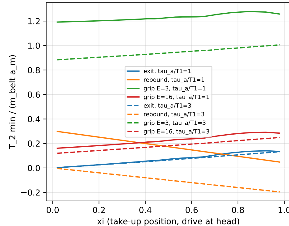
(d) Min. T_2 , drive at head, \gamma = 2 , \rho = 1
