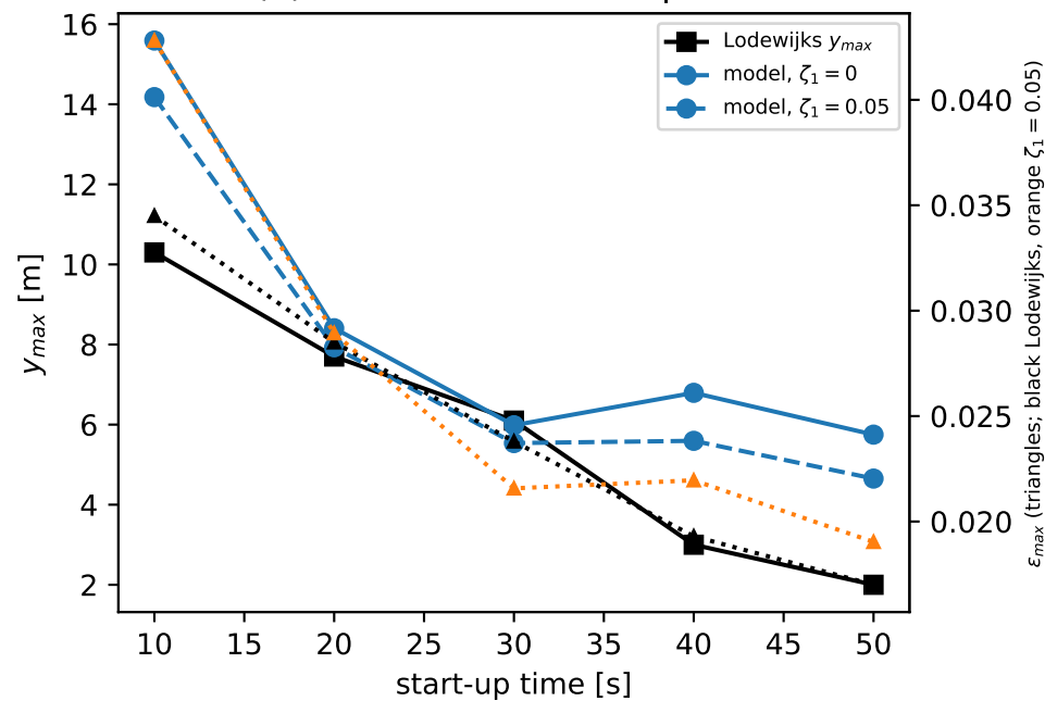
(d) linear offset, start-up time
