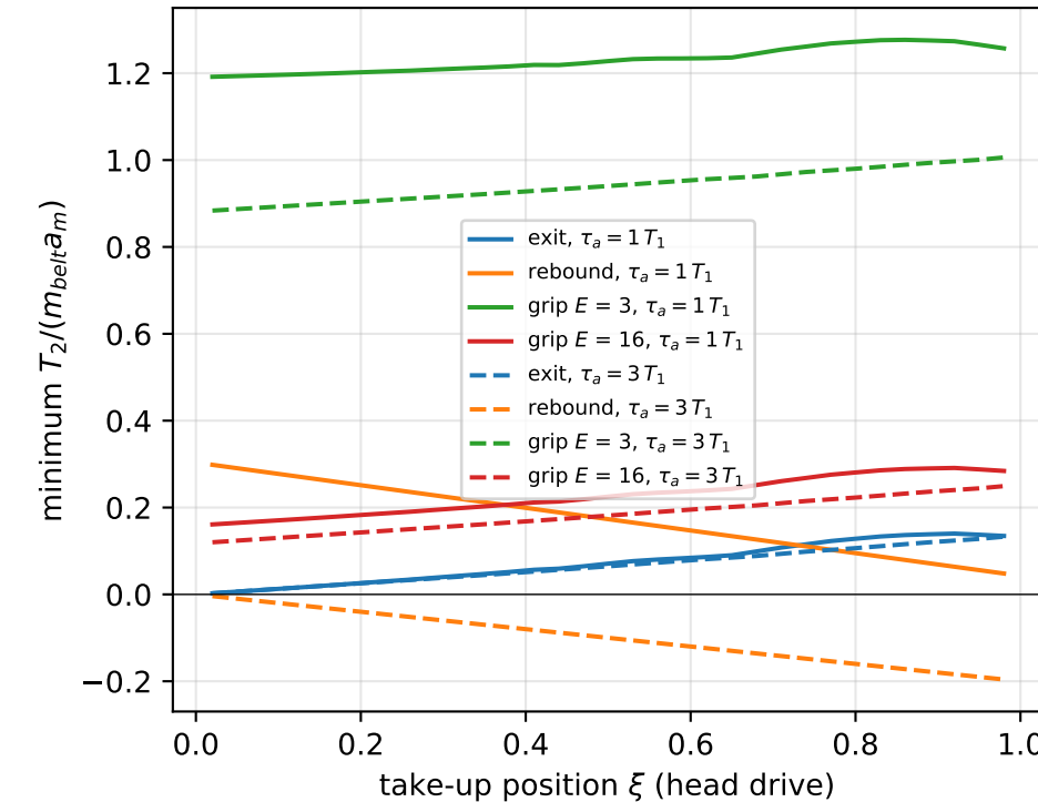
(d) minimum T_2 , head drive, \gamma = 2, \rho = 1
