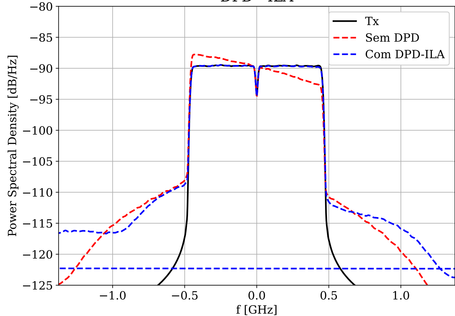
DPD - ILA
