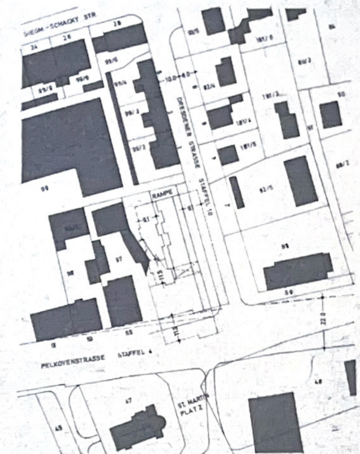
LAGEPLAN M 1:1000
