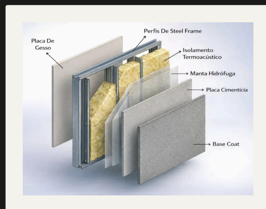
DIAGRAMA DAS CAMADAS DE UMA PAREDE EM LIGHT STEEL FRAME
