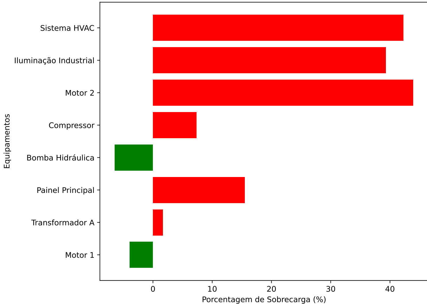
Porcentagem de Sobrecarga por Equipamento
