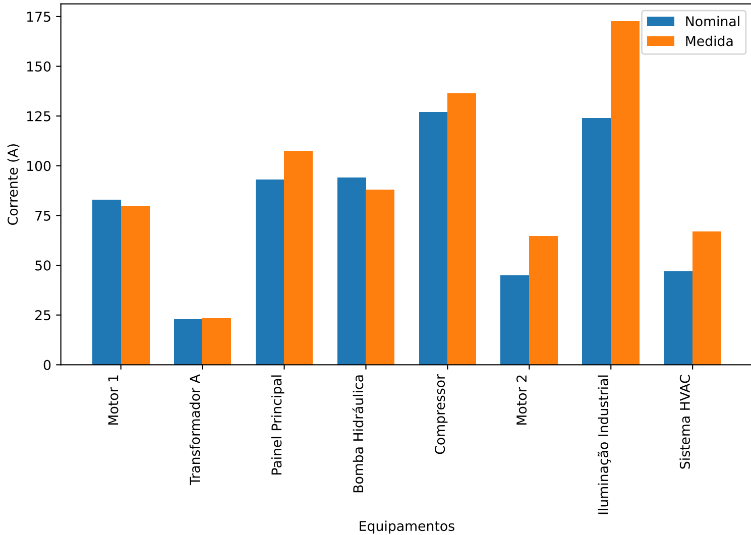
Corrente Nominal vs Corrente Medida
