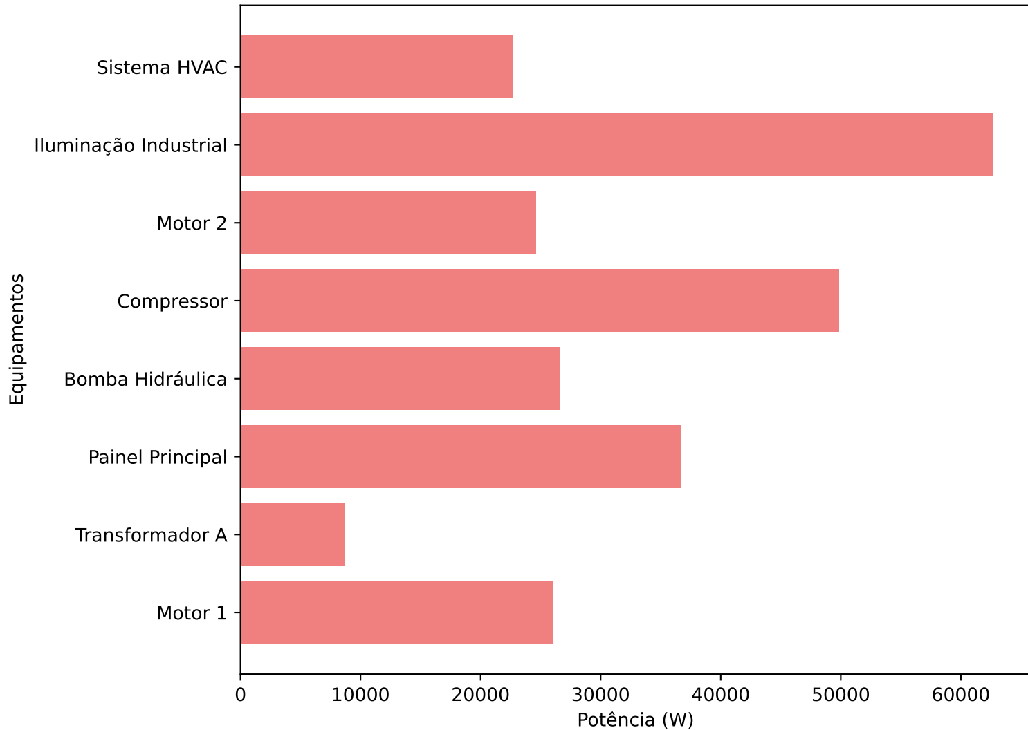
Potência dos Equipamentos
