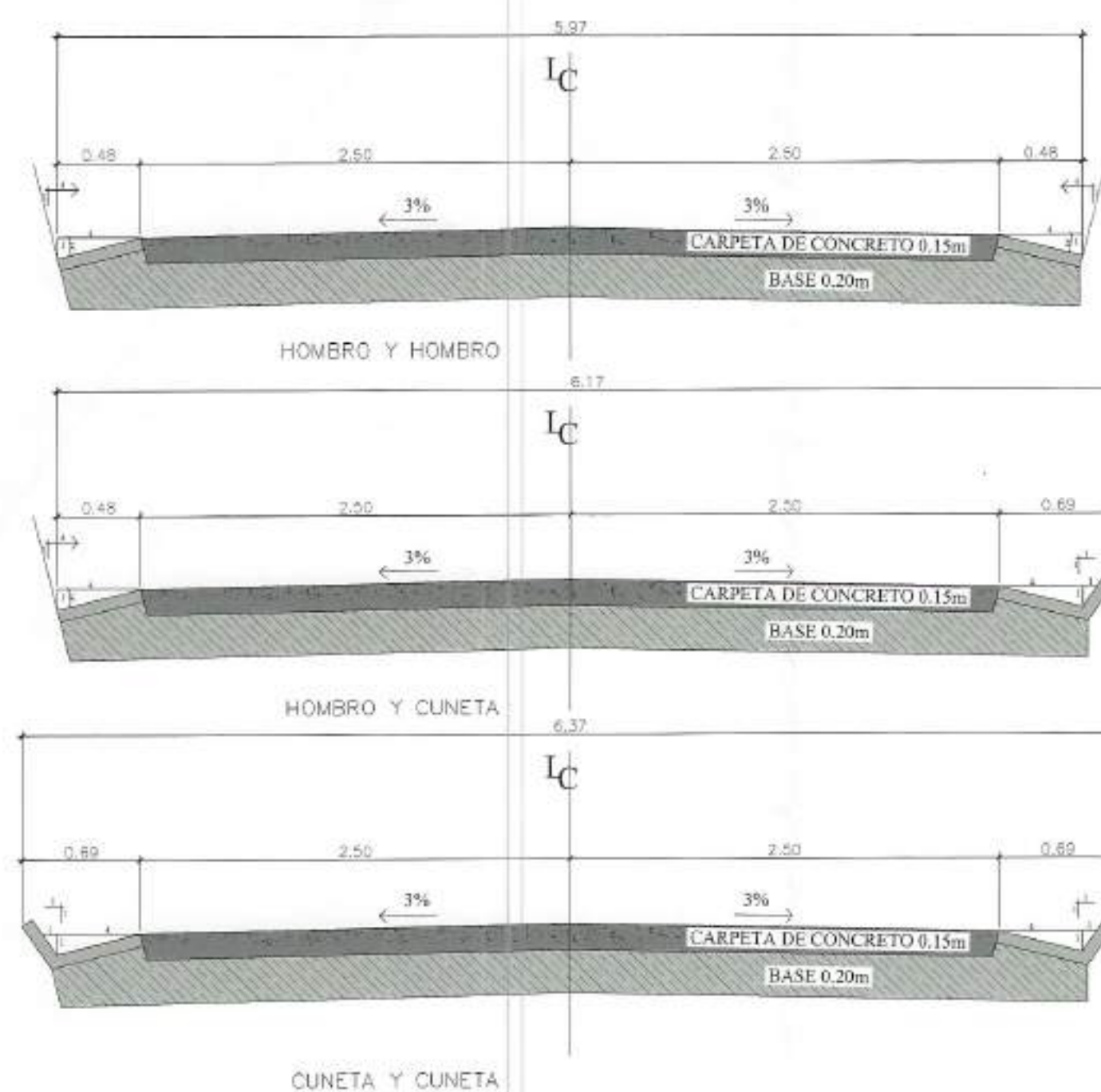
SECCIONES TÍPICAS DE CARRILES
