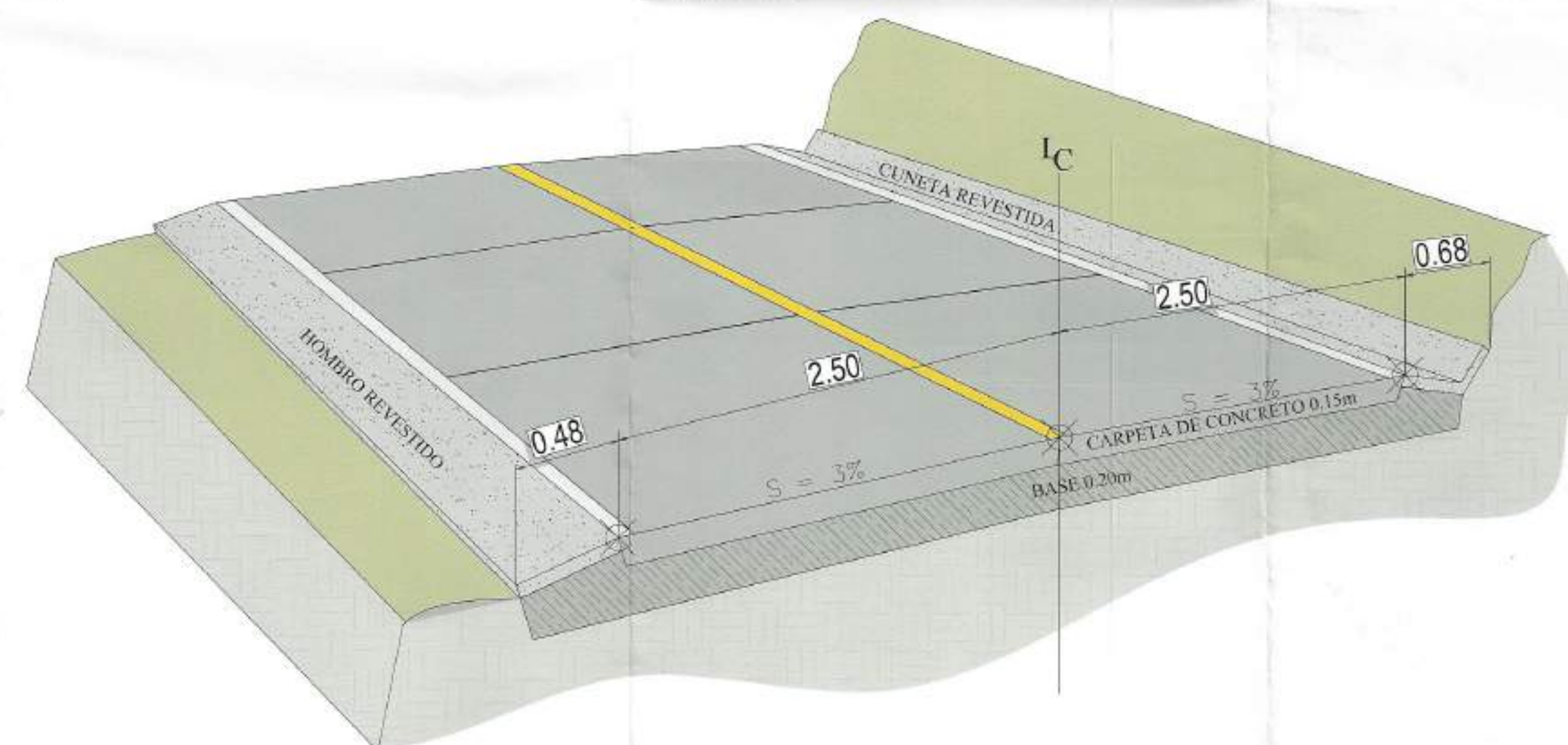
ISOMETRICO DE SECCION TIPICA
