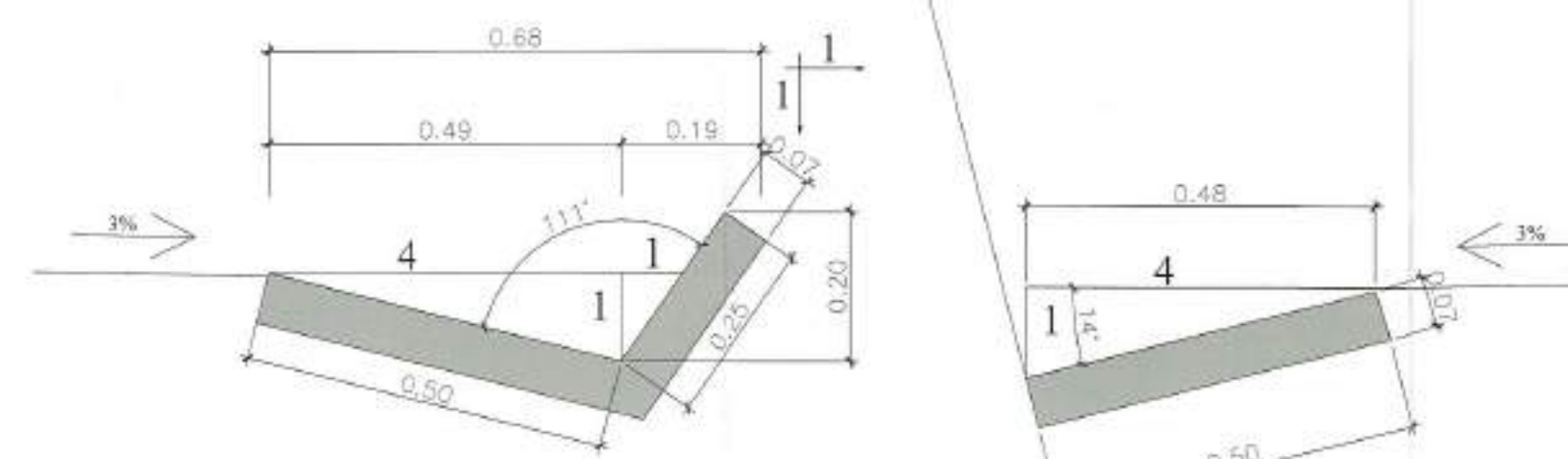
DETALLE DE CUNETA Y HOMBRO
