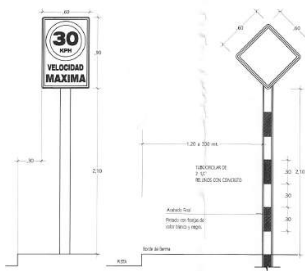
UBICACION DE SEÑALES VERTICALES CON RELACION AL BORDE Y NIVEL DE LA VIA Escala 1:25
