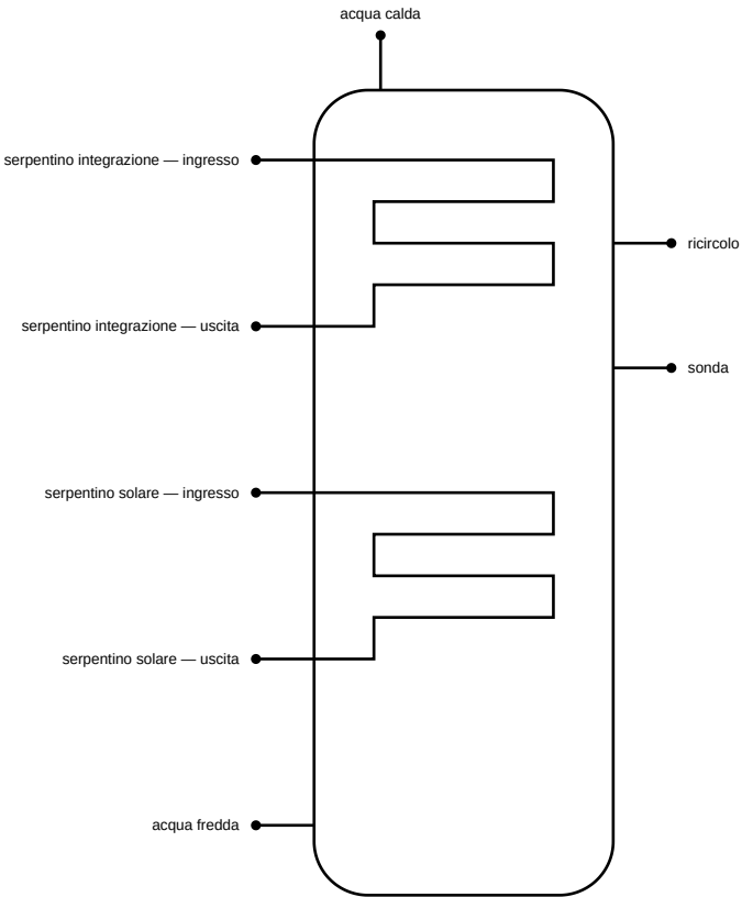
Bollitore ACS a due serpentini
