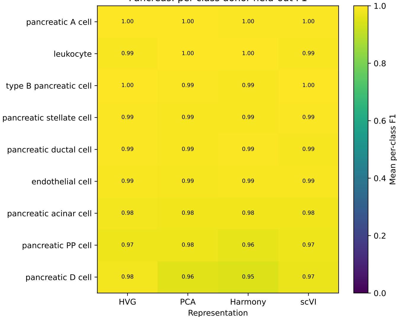
Pancreas: per-class donor-held-out F1
