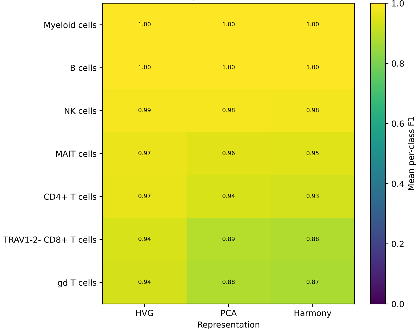
Blood Atlas: per-class donor-held-out F1
