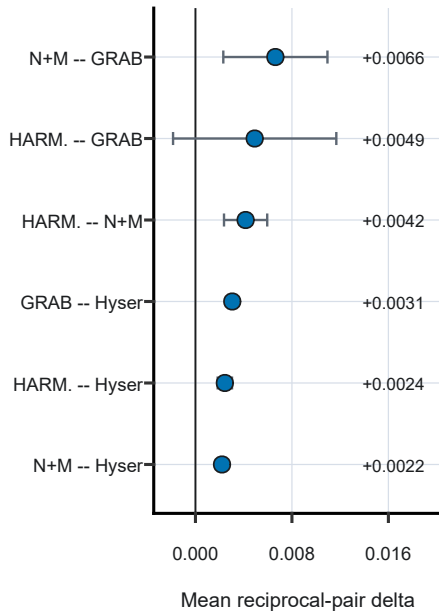
B. Reciprocal-pair CKA
