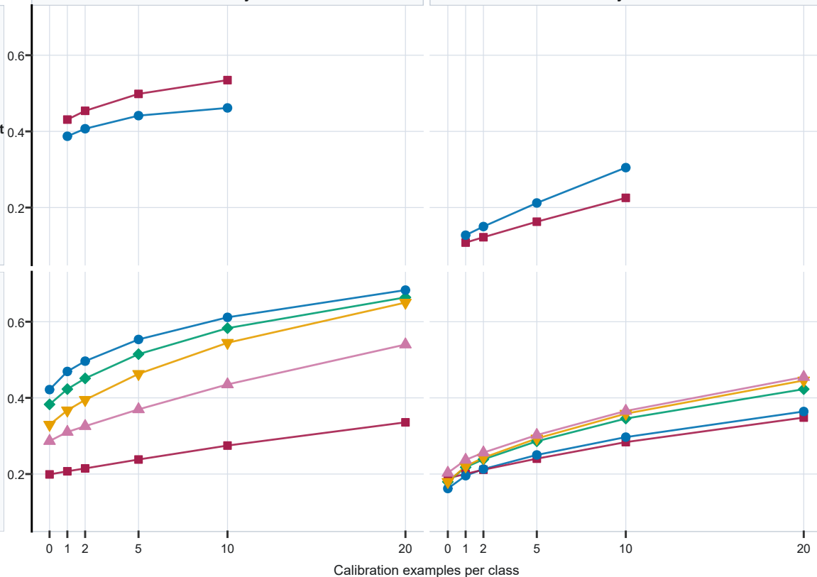
GRABMyo
