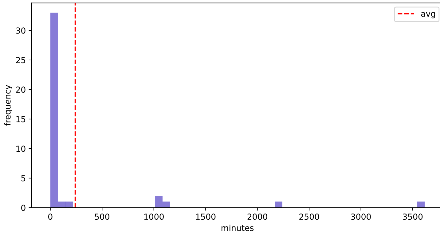
BPIC2012 - W_Beoordelen fraude (Avg 240.50 min, Std 702.67 min)
