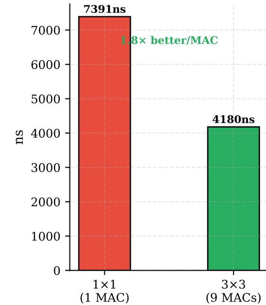
Latency per MAC
