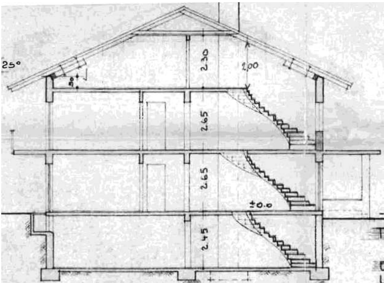
Schnitt westlicher Teil
