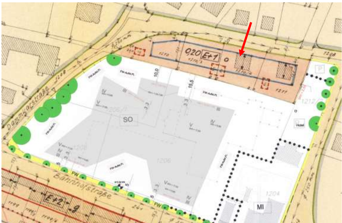
Auszug Bebauungsplan Nr. 5 mit Bebauungsplan Nr. 42 von 2011; Einfügen Bebauungsplan Nr. 42 (weißer Hintergrund) und graue Färbung des Bauraums durch den Sachverständigen;
