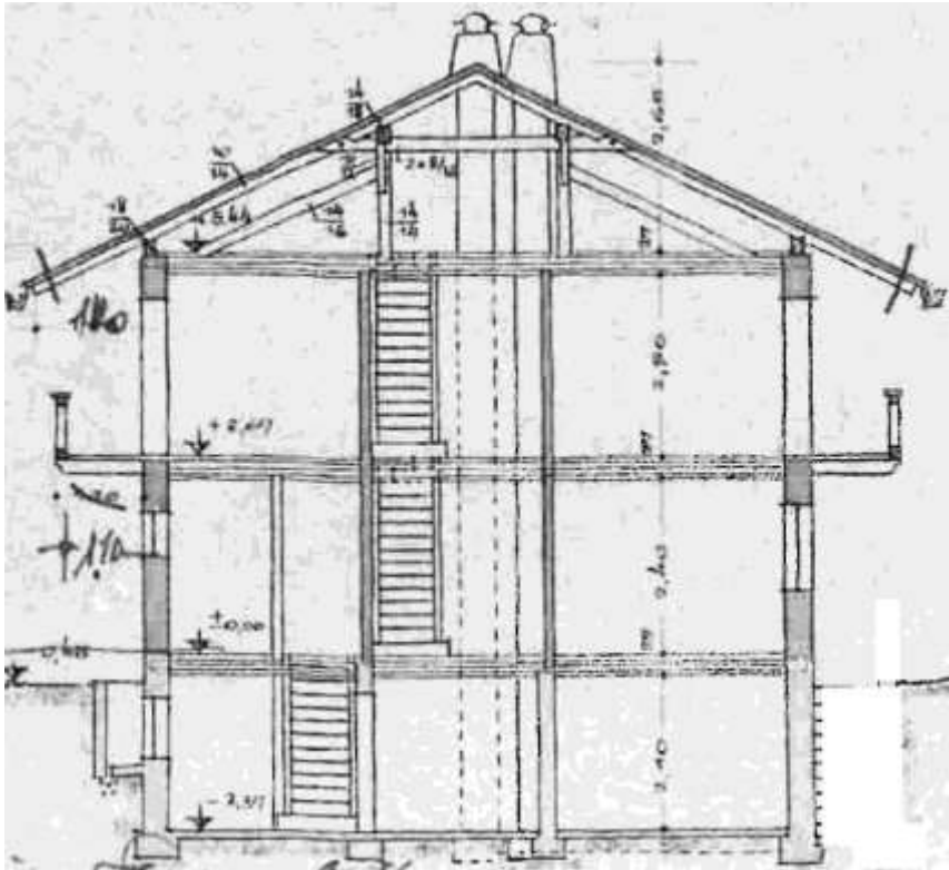
Schnitt östlicher Teil (Treppe nicht aktuell)
