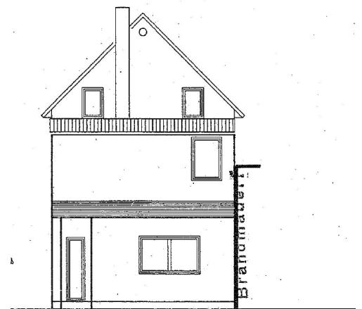
Gartenansicht ( Westen )
