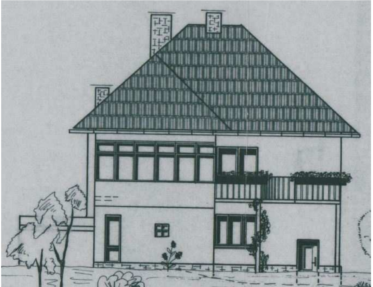
Westansicht aus der Bauakte von 1983
