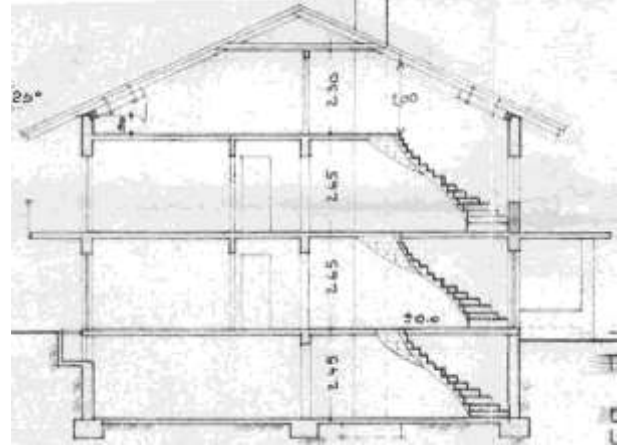
Schnitt
