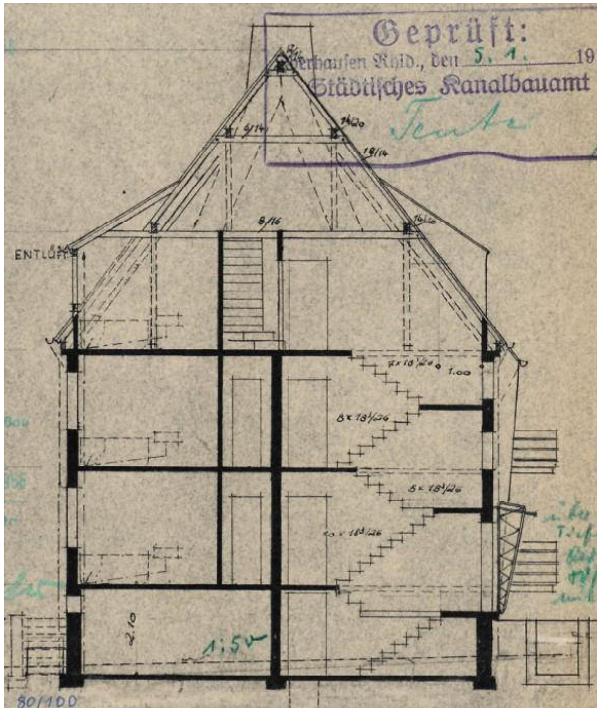
Schnitt gemäß Baugenehmigung von 1957
