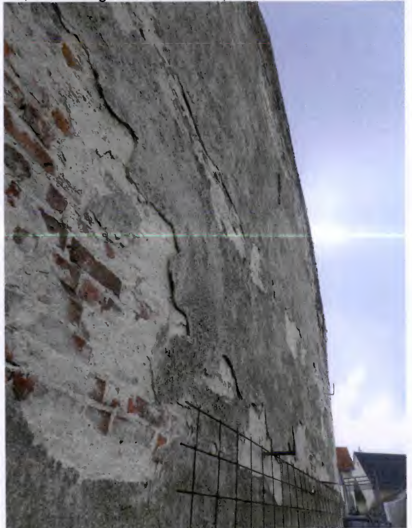
Bild 8: Scheune, Schäden am Außenputz
