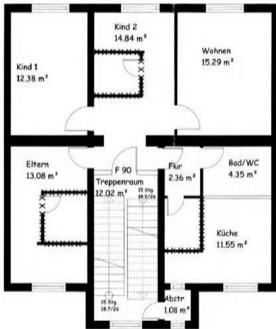
Grundriss 1. – 3. Obergeschoss (2004)
