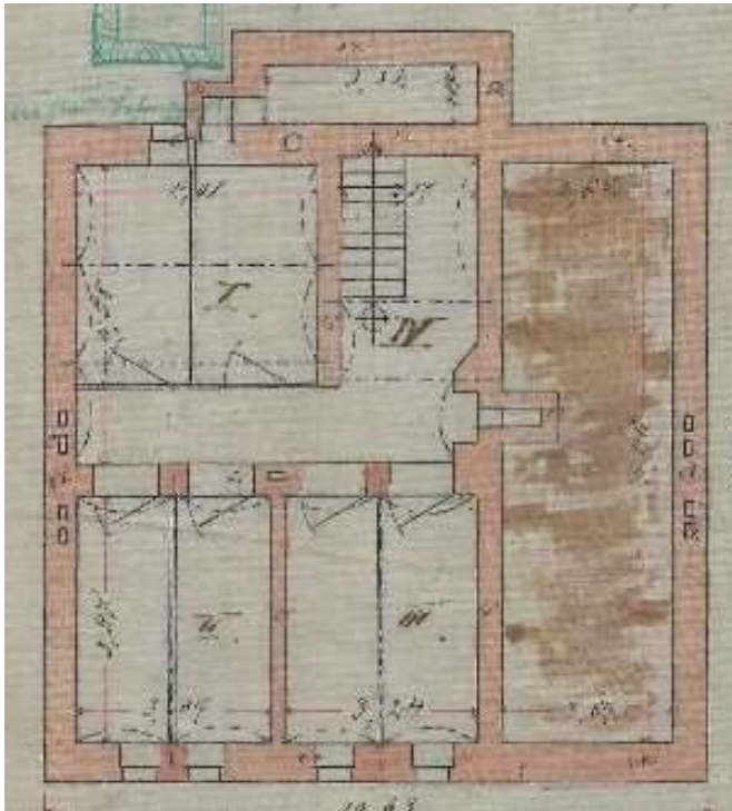
Grundriss Kellergeschoss (1901)
