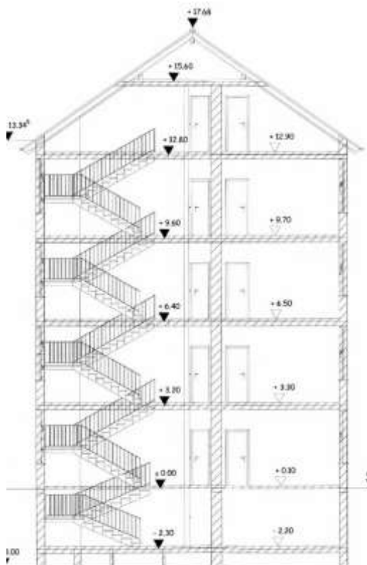
Schnitt A-A (2004)
