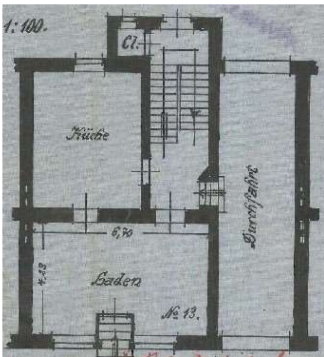
Grundriss Erdgeschoss (1928)
