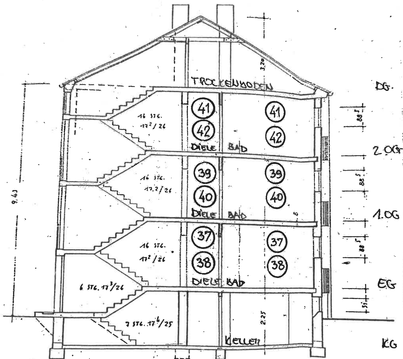
SCHNITT HAUS NR. 104
