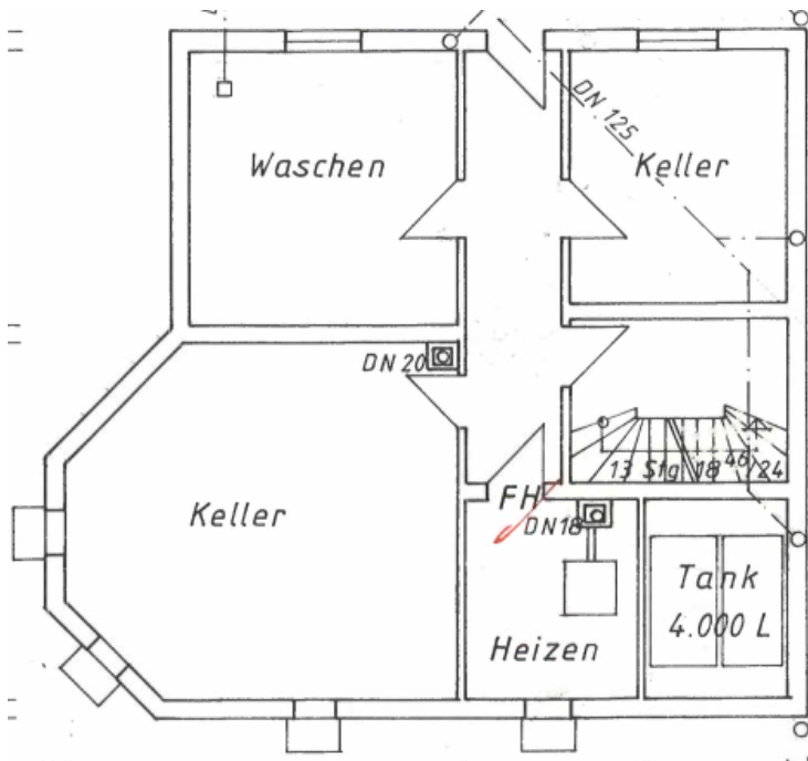
Kellergeschossgrundriss des Wohnhauses
