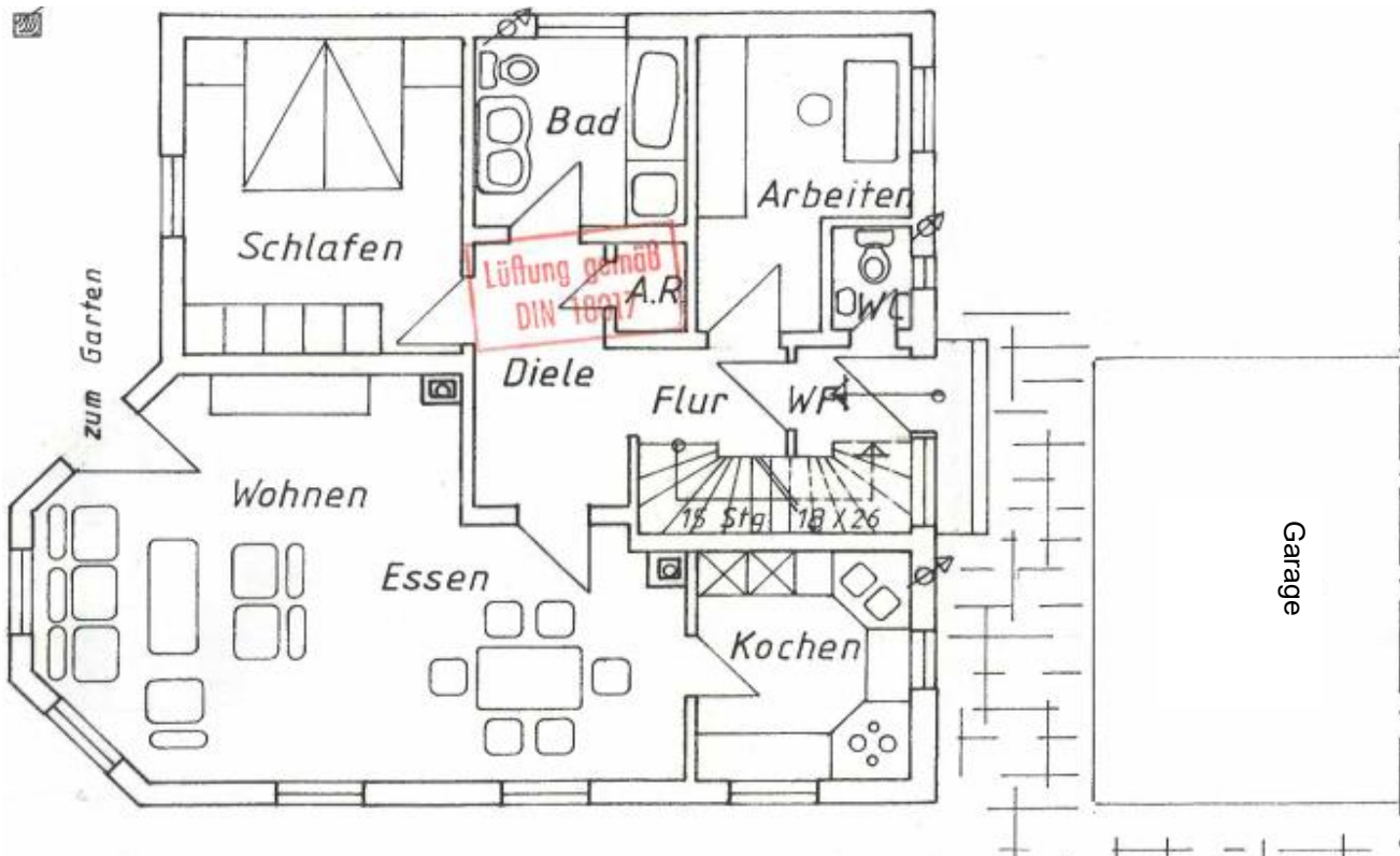
Erdgeschossgrundriss
