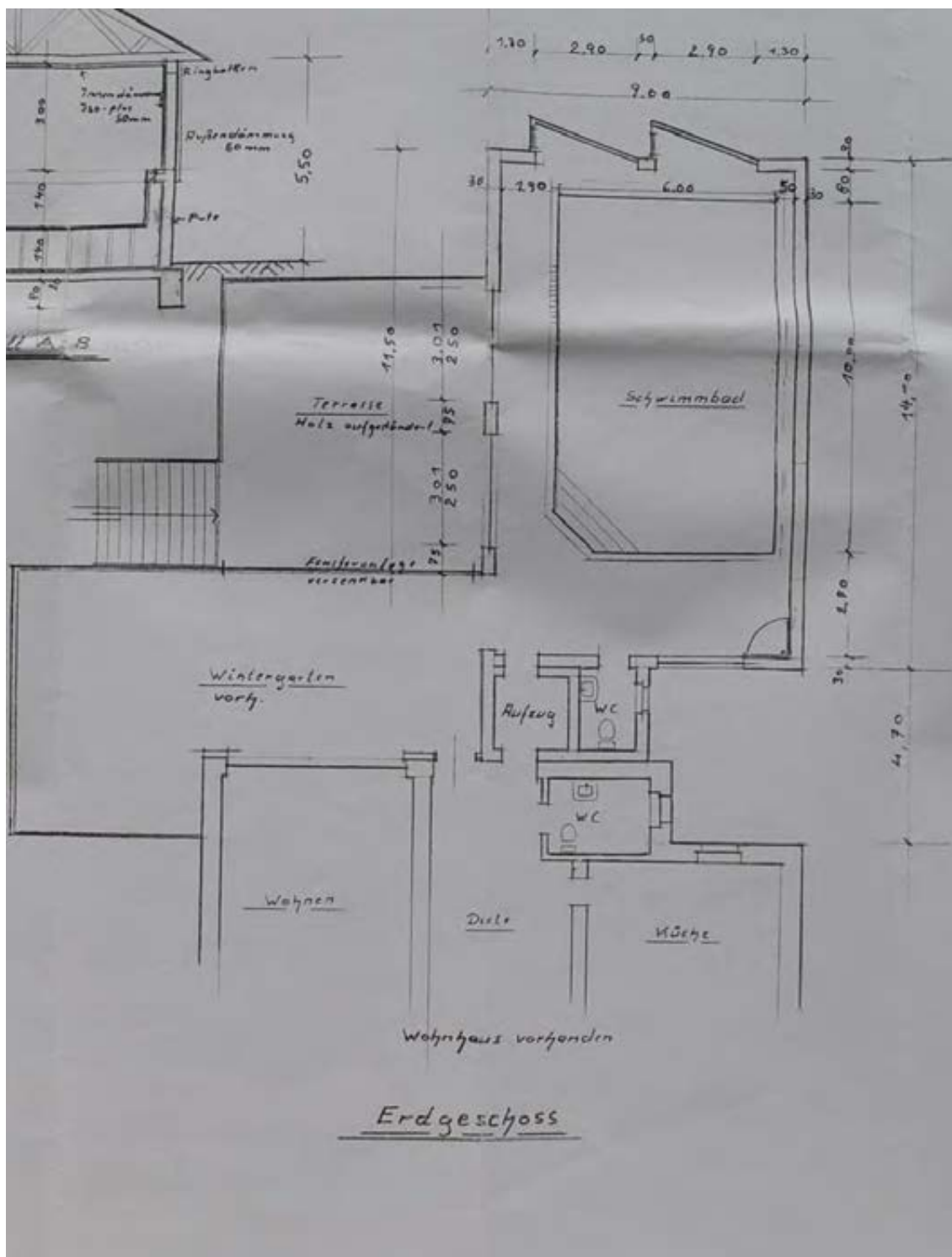
Grundriss Erdgeschoss (Schwimmbad)
