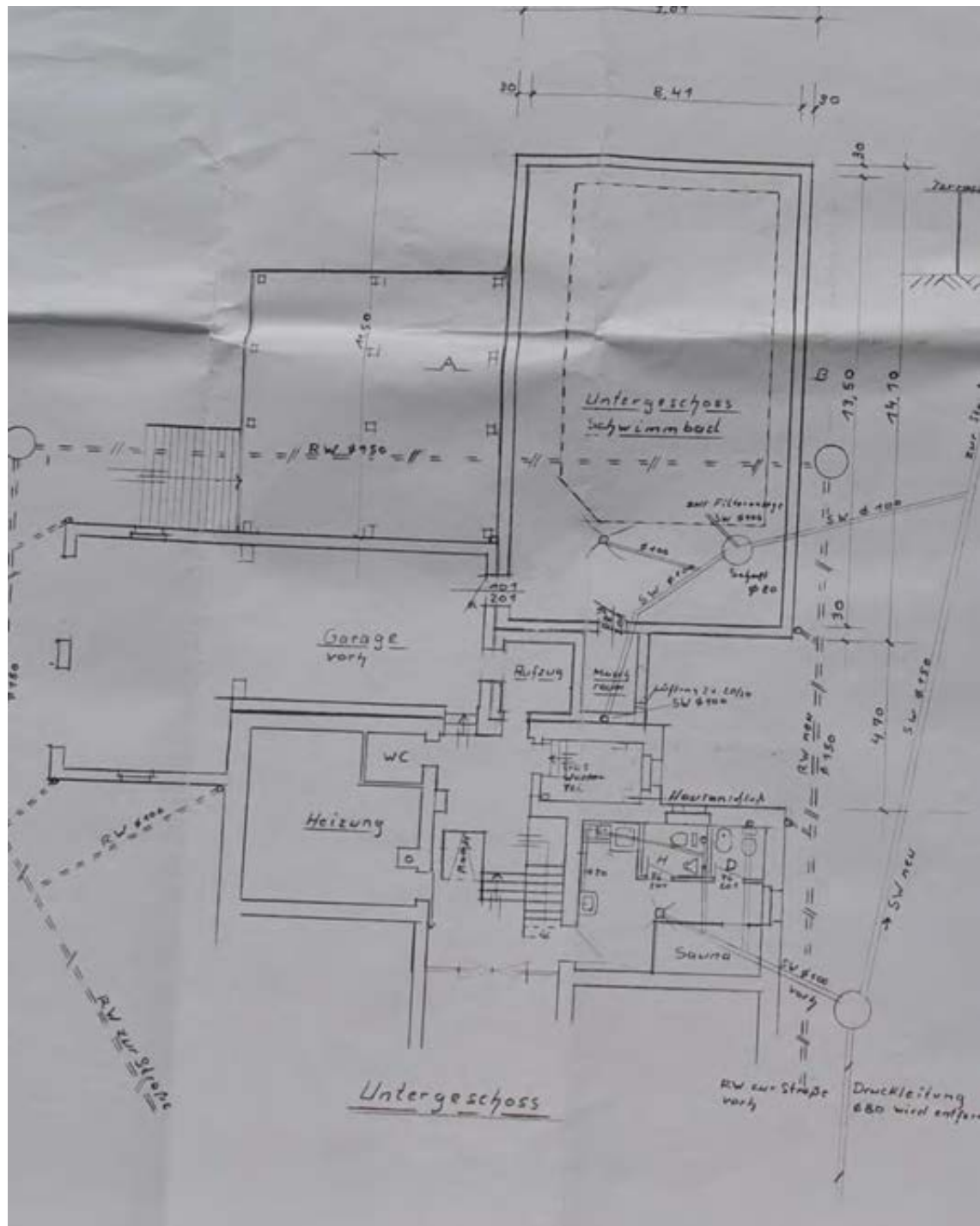
Grundriss Kellergeschoss (Schwimmhalle)
