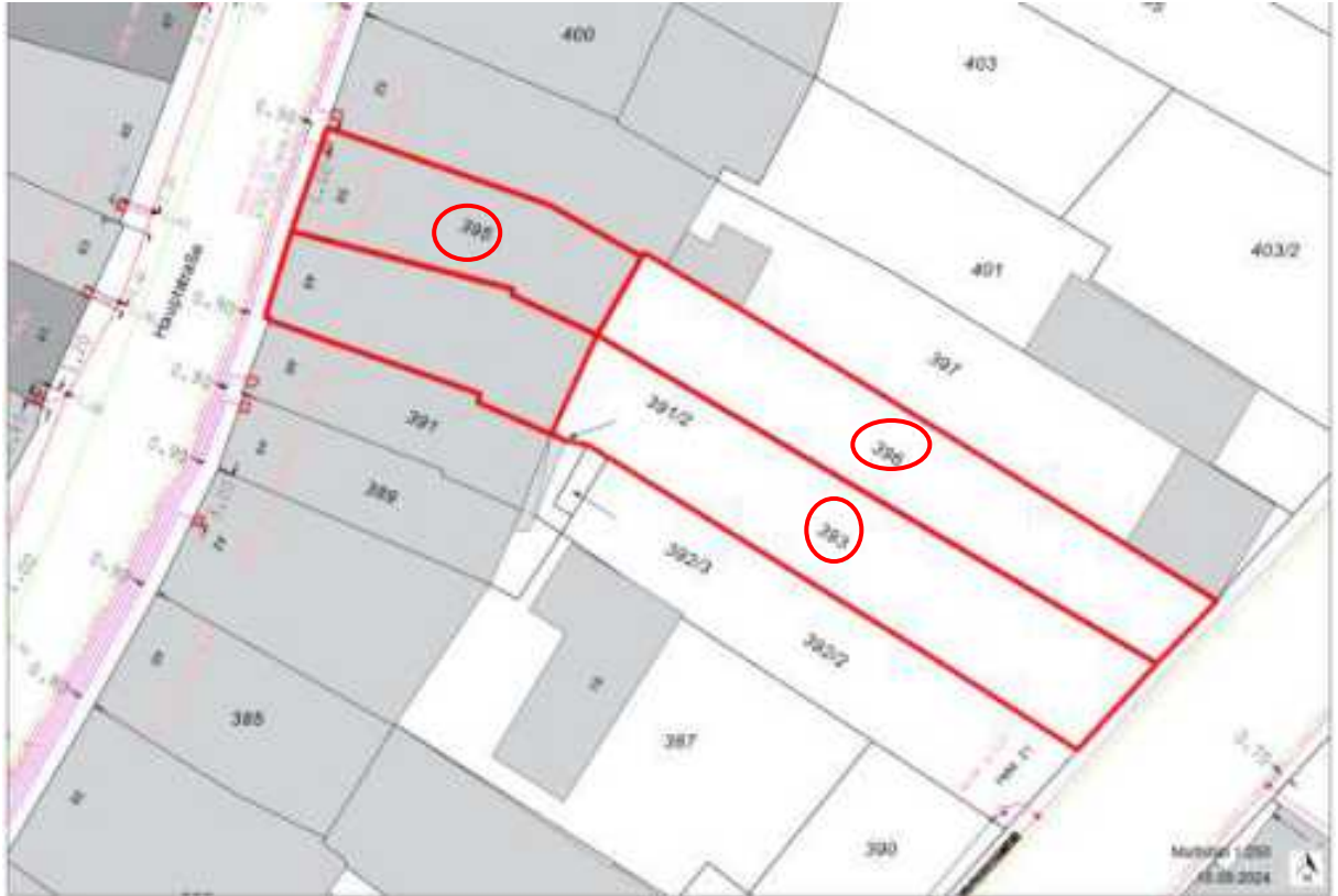
Auszug aus dem Spartenplan - Strom (kein Maßstab!)
