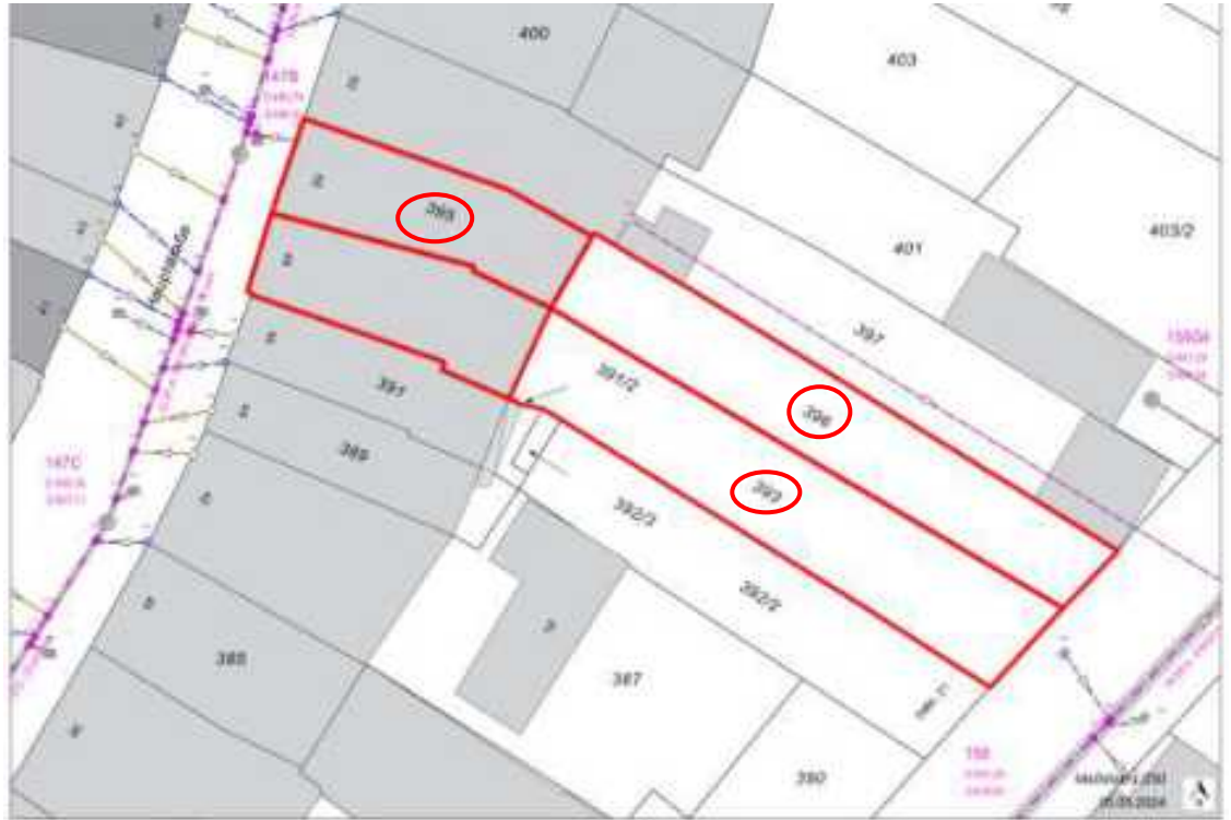
Auszug aus dem Spartenplan - Kanal (kein Maßstab!)
