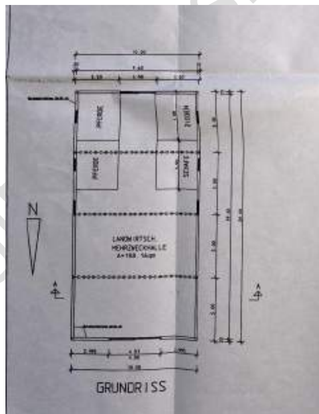
Mehrzweckhalle
