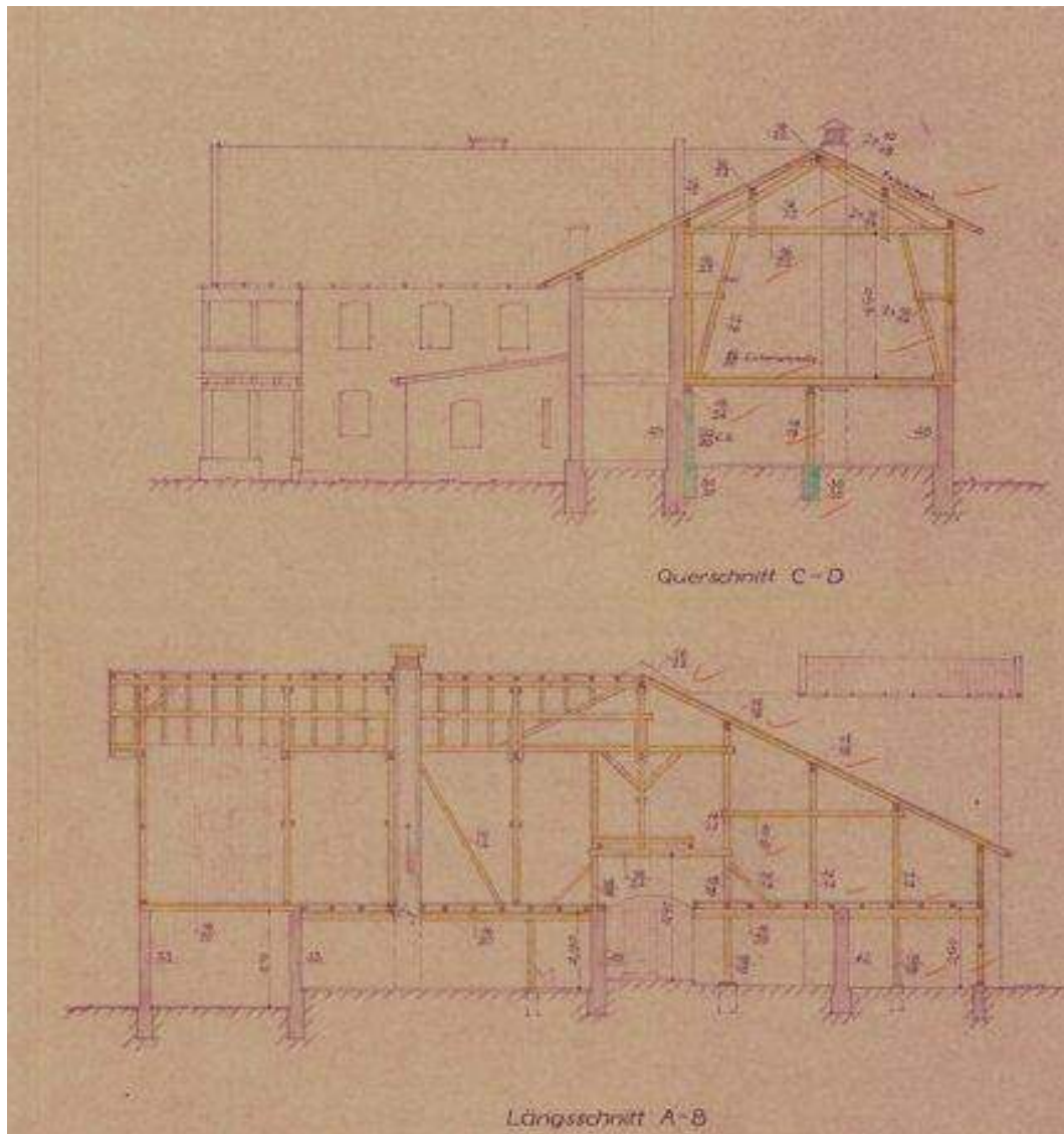
Wohnhaus/Stall Tenne
