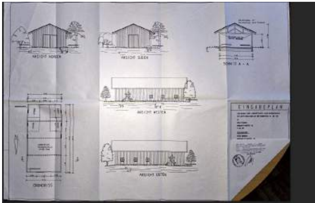
Mehrzweckhalle
