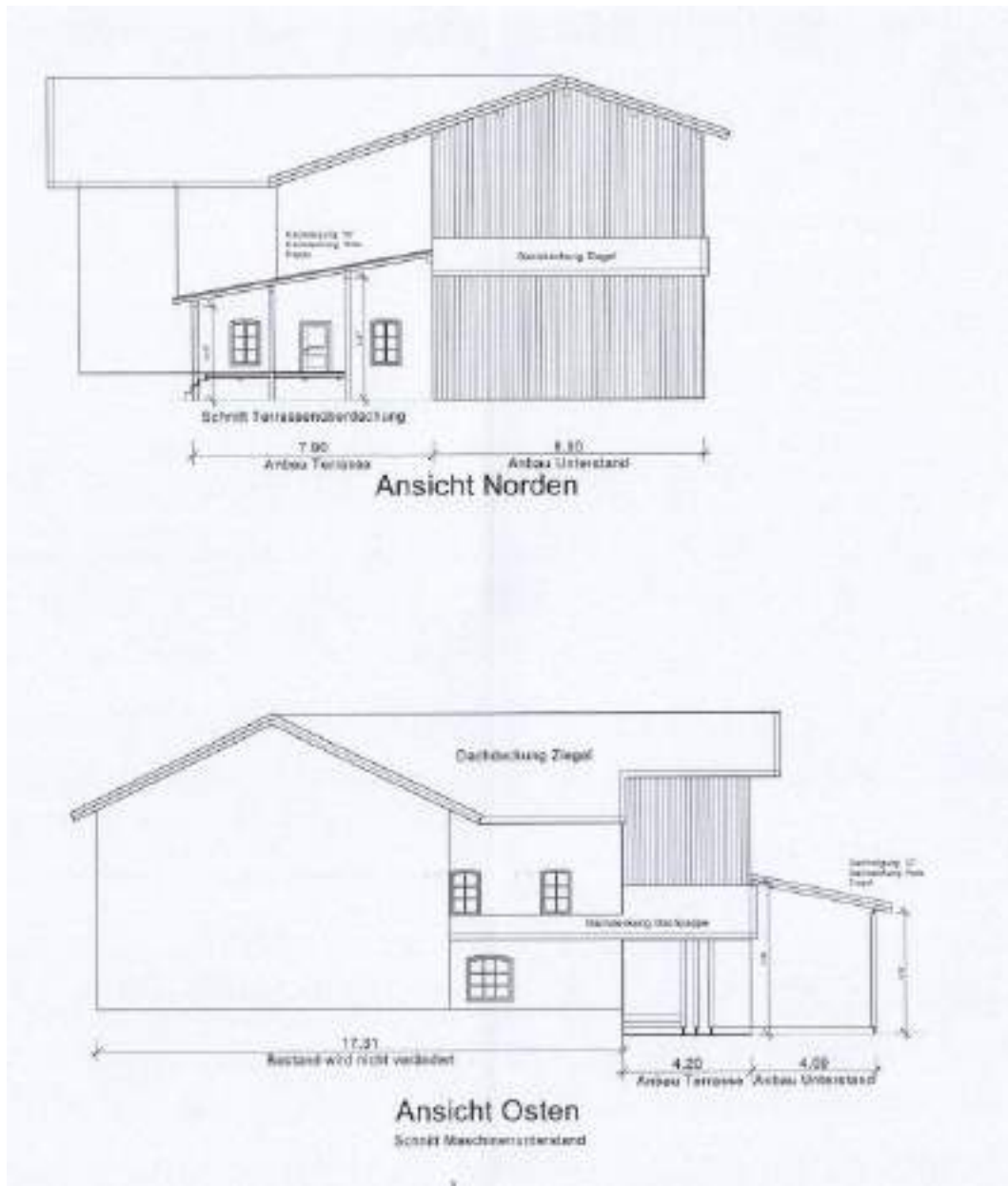
Wohnhaus Anbau
