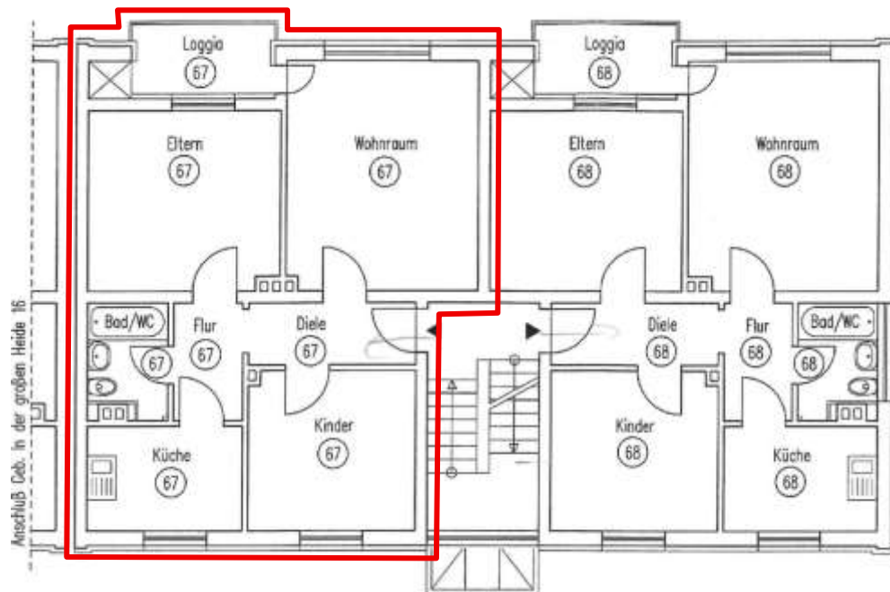
Grundriss 1. Obergeschoss
