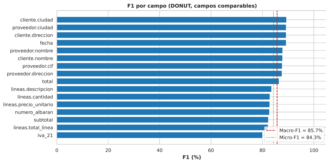
b) Rendimiento de DONUT
