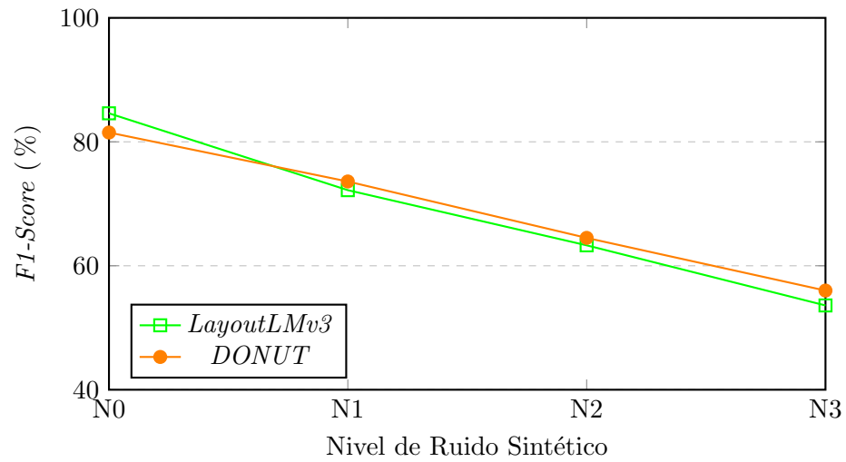
Figura 16: Evolución consolidada del rendimiento global frente a la degradación visual.
