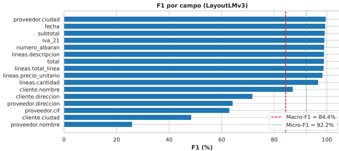
a) Rendimiento de LayoutLMv3
