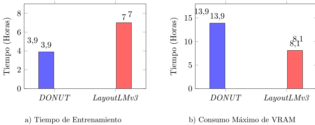
Figura 18: Comparativa de costes computacionales durante la fase de adaptación al dominio (entrenamiento).
