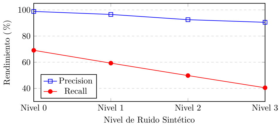
Figura 14: Evolución de la precisión y el Recall frente a la degradación visual en el modelo DONUT .
