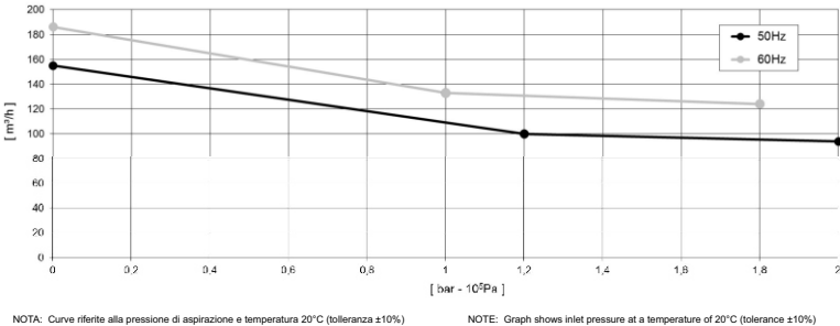
NOTA: Curve riferite alla pressione di aspirazione e temperatura 20°C (tolleranza ±10%) NOTE: Graph shows inlet pressure at a temperature of 20°C (tolerance ±10%)
